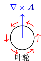
(a) 有旋场 \nabla \times \mathbf{A} \neq \mathbf{0} 叶轮旋转
