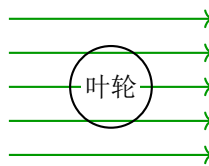
(b) 无旋场 \nabla \times \mathbf{A} = \mathbf{0} 叶轮不转
