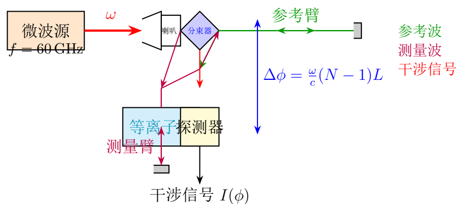
图 12.2: 微波干涉仪光路示意图。微波源经分束器分为参考臂和测量臂, 测量臂穿过等离子体后产生相位移 \Delta\phi , 两束波在分束器处重新汇合产生干涉, 由探测器记录。
