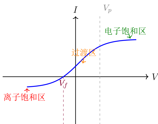
图 12.1: 朗缪尔探针典型 I - V 特性曲线。横轴为探针电压 V ，纵轴为收集电流 I 。 V_p 为等离子体电位， V_f 为悬浮电位（净电流 I = 0 处）。曲线分为三个主要区域：离子饱和区 ( V \ll V_p )、过渡区 ( V_f \lesssim V \lesssim V_p ) 和电子饱和区 ( V \gg V_p )。
