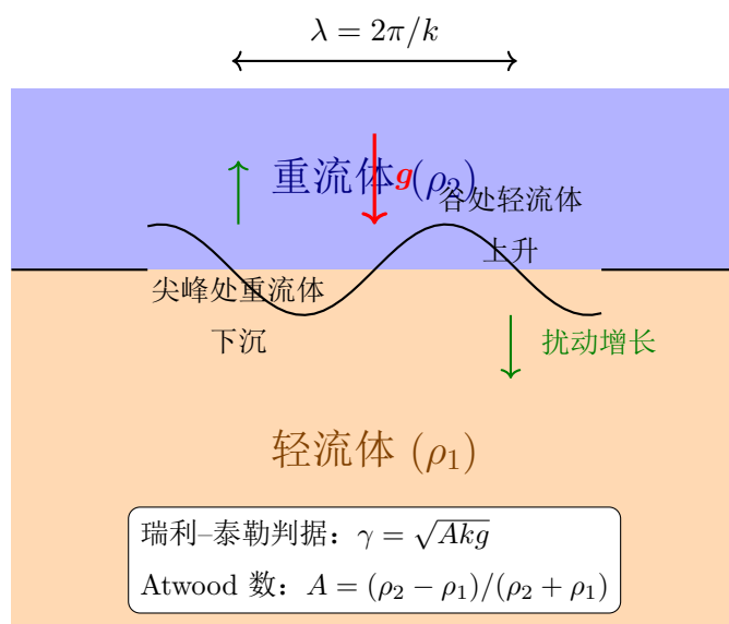
图 9.3: 瑞利-泰勒不稳定性物理图像。重流体在轻流体上方，在有效重力 g 作用下，界面扰动（尖峰和谷）被放大。尖峰处重流体下沉，谷处轻流体上升，形成反馈循环，扰动指数增长。
