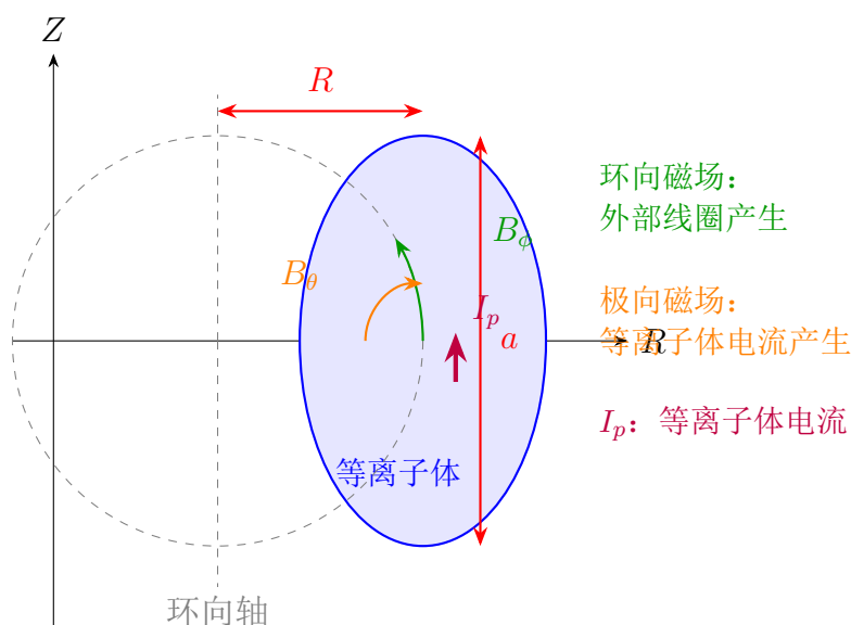
图 10.1: 托卡马克位形示意图 ( R 为大半径, a 为小半径, B_\phi 为环向磁场, B_\theta 为极向磁场, I_p 为等离子体电流)。
