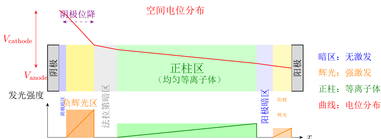
图 11.1: DC 辉光放电空间结构示意图。从阴极到阳极依次可见: 阴极暗区、负辉光区 (最亮)、法拉第暗区、正柱区 (均匀等离子体)、阳极暗区、阳极辉光。上图红线为空间电位分布, 下方柱状图示意发光强度。
