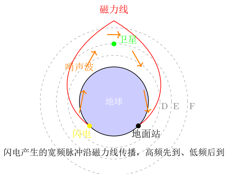
图 6.2: 哨声波传播路径示意图。闪电激发的电磁脉冲沿地球磁力线传播，在电离层 D/E/F 层中穿过，到达另一半球的地面站。
