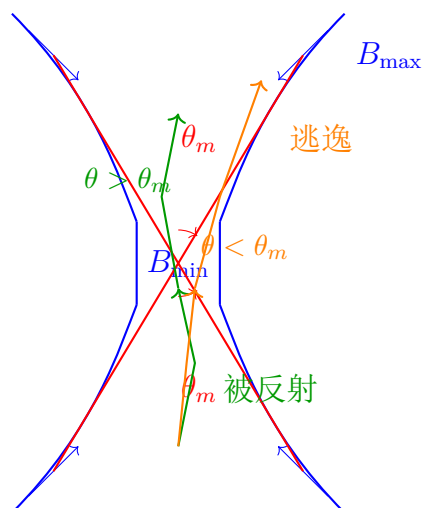
图 3.2: 磁镜损失锥示意图。在磁镜喉部 B_{\max} 处，若粒子投掷角 \theta < \theta_m ，则 v_{\perp}^2 不足以将平行动能完全转化为垂直动能，粒子将穿过磁镜逃逸。
