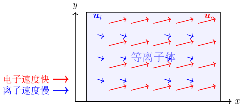
图 4.1: 双流体模型示意图。电子和离子作为两种独立的流体，可以具有不同的宏观流速 u_e 和 u_i 。由于 m_e \ll m_i ，电子的响应远快于离子。
