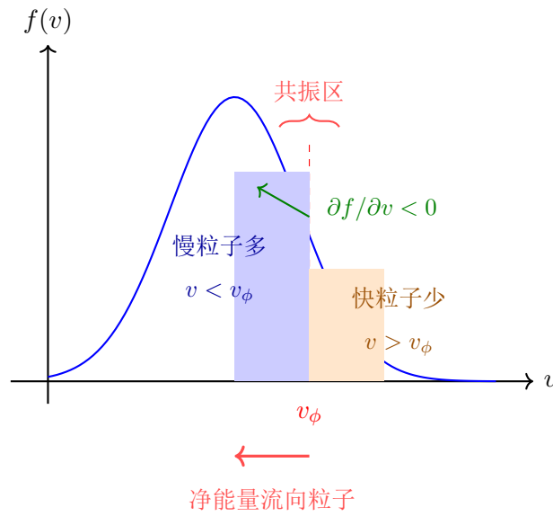
图 7.1: Landau 阻尼的共振粒子示意图。在相速度 v_\phi 附近，速度略小于 v_\phi 的粒子比速度略大于 v_\phi 的粒子多 ( \partial f_0 / \partial v < 0 )，导致净能量从波流向粒子，波被阻尼。
