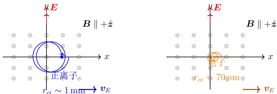
图 3.1: E \times B 漂移的摆线轨迹。磁场垂直纸面向外，电场沿 +y 方向。正离子逆时针回旋，电子顺时针回旋，但两者漂移方向相同（均沿 +x ）。
