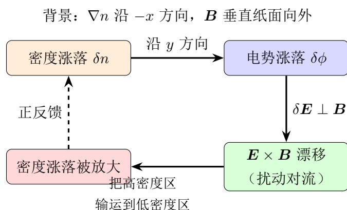
图 9.1: 漂移波不稳定性的正反馈回路。密度梯度 (沿 -x 方向) 中的密度涨落产生电势涨落, 电势涨落的 \mathbf{E} \times \mathbf{B} 漂移把高密度等离子体输运到低密度区, 进一步放大密度涨落——扰动指数增长。磁场 \mathbf{B} 垂直纸面向外。
