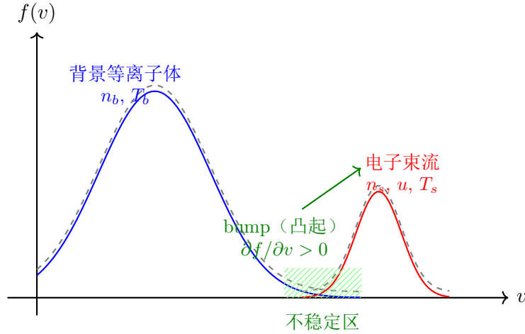
图 7.2: bump-on-tail 速度分布函数示意图。蓝色宽峰为背景热电子，红色窄峰为漂移电子束流。在两峰之间的“尾部”区域形成凸起 (bump)，对应 \partial f/\partial v > 0 ，驱动 Langmuir 波不稳定性增长。
