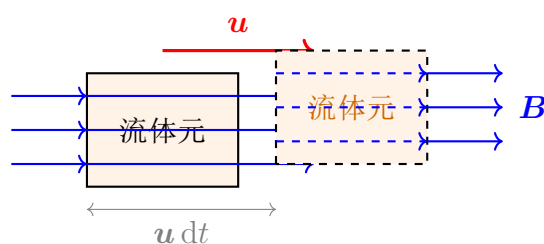
图 5.1: 磁力线冻结示意图。在理想导电流体 ( R_m \gg 1 ) 中, 磁通量随流体元守恒, 磁力线仿佛被”冻结”在流体中。
