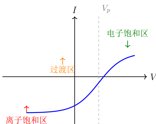
图 12.1: 朗缪尔探针典型 I - V 特性曲线。横轴为探针电压 V ，纵轴为收集电流 I 。 V_p 为等离子体电位。曲线分为三个主要区域：离子饱和区 ( V \ll V_p )、过渡区 ( V \approx V_p ) 和电子饱和区 ( V \gg V_p )。
