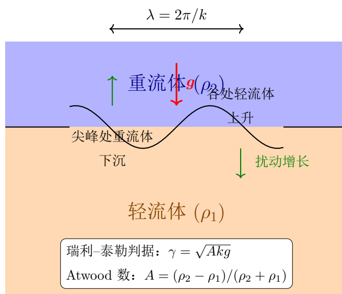
图 9.2: 瑞利-泰勒不稳定性物理图像。重流体在轻流体上方，在有效重力 g 作用下，界面扰动（尖峰和谷）被放大。尖峰处重流体下沉，谷处轻流体上升，形成反馈循环，扰动指数增长。
