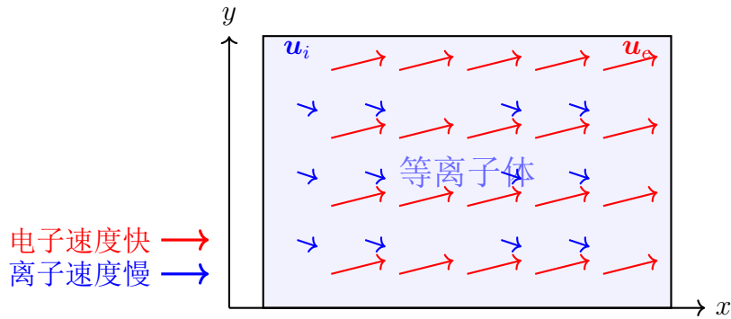
图 4.1: 双流体模型示意图。电子和离子作为两种独立的流体，可以具有不同的宏观流速 \mathbf{u}_e 和 \mathbf{u}_i 。由于 m_e \ll m_i ，电子的响应远快于离子。
