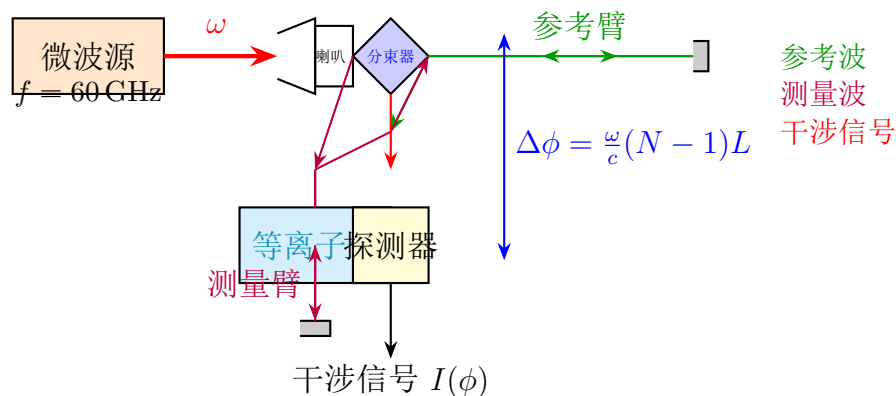
图 12.2 微波干涉仪光路示意图。微波源经分束器分为参考臂和测量臂，测量臂穿过等离子体后产生相移 \Delta\phi ，两束波在分束器处重新汇合产生干涉，由探测器记录。
