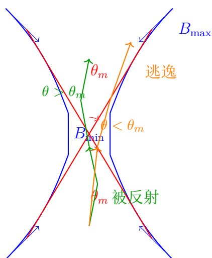
图 3.2 磁镜损失锥示意图。粒子在强场区被反射的条件是 \sin^2 \theta \geq 1/R_m ：投掷角 \theta > \theta_m 的粒子垂直速度分量足够大，向镜点运动时 v_\perp 随 B 增大而增大，最终 v_\parallel 降为零并被反射；而 \theta < \theta_m 的粒子 v_\perp 太小，磁矩不变性不足以在其抵达镜点前反转 v_\parallel ，因而穿过磁镜逃逸。这些 \theta < \theta_m 的方向构成损失锥。
