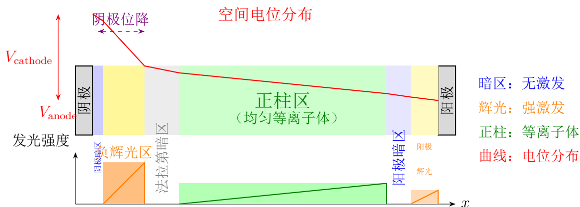
图 11.1 DC 辉光放电空间结构示意图。从阴极到阳极依次可见：阴极暗区、负辉光区（最亮）、法拉第暗区、正柱区（均匀等离子体）、阳极暗区、阳极辉光。上图红线为空间电位分布，下方柱状图示意发光强度。
