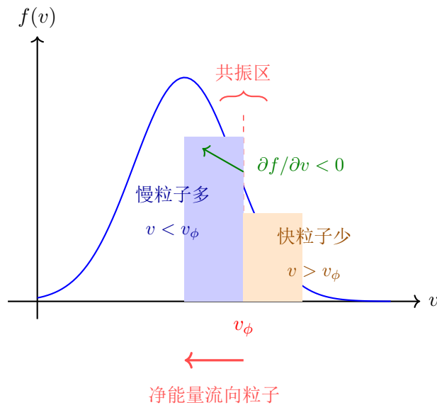
图 7.1 Landau 阻尼的共振粒子示意图。在相速度 v_\phi 附近，速度略小于 v_\phi 的粒子比速度略大于 v_\phi 的粒子多 ( \partial f_0 / \partial v < 0 )，导致净能量从波流向粒子，波被阻尼。
