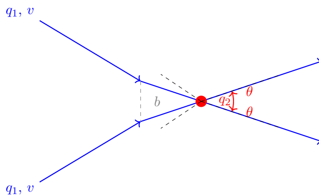
图 8.1 库仑碰撞小角度散射示意图。带电粒子 q_1 以速度 v 经过靶粒子 q_2 附近，由于长程库仑力，轨迹发生轻微偏折。偏转角 \theta 很小，但远距离碰撞频繁发生，累积效应主导了动量输运。
