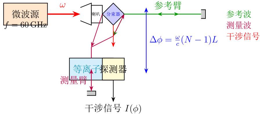
图 12.2 微波干涉仪光路示意图。微波源经分束器分为参考臂和测量臂，测量臂穿过等离子体后产生相位移动 \Delta\phi ，两束波在分束器处重新汇合产生干涉，由探测器记录。
