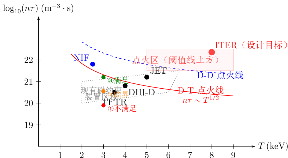
图 10.2 Lawson 参数空间图: n\tau 对温度 T 的依赖关系。图中标注了若干代表性装置 (TFTR、JET、DIII-D、NIF) 以及 ITER 的设计目标。判据方向: 固定温度时, 必须 n\tau 高于点火线才满足点火条件, 所以能量自持区在点火线上方 (图中红色阴影区); 线下方为不满足区。三点示意: ①在阈值线下 (不满足)、②恰在线上 (临界)、③在线上方 (满足)。
