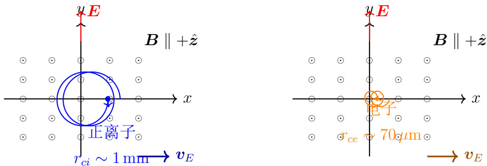
图 3.1 E \times B 漂移的摆线轨迹。磁场垂直纸面向外 ( +\hat{z} ), 电场沿 +y 方向。取初速度方向向右: 正电荷受力 q\mathbf{v} \times \mathbf{B} 指向下方, 故正离子顺时针回旋; 电子受力反向, 故电子逆时针回旋。两者回旋方向相反, 但漂移方向相同 (均沿 +\hat{x} , 因 \mathbf{v}_E = \mathbf{E} \times \mathbf{B}/B^2 与电荷符号无关)。
