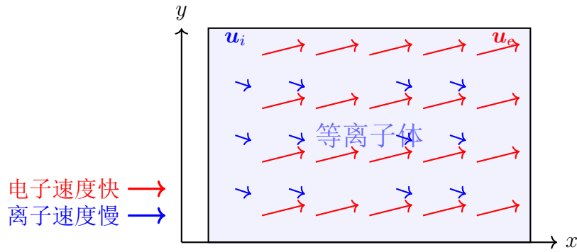
图 4.1 双流模型示意图。电子和离子作为两种独立的流体，可以具有不同的宏观流速 u_e 和 u_i 。由于 m_e \ll m_i ，电子的响应远快于离子。
