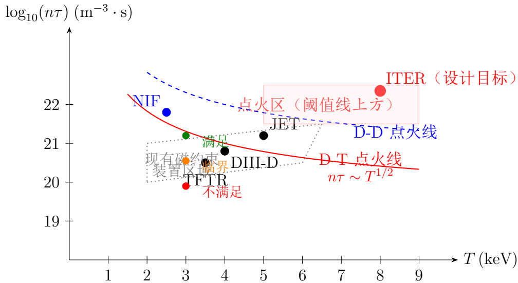
图 10.2 Lawson 参数空间图: n\tau 对温度 T 的依赖关系。图中标注了若干代表性装置 (TFTR、JET、DIII-D、NIF) 以及 ITER 的设计目标。判据方向: 固定温度时, 必须 n\tau 高于点火线才满足点火条件, 所以能量自持区在点火线上方 (图中红色阴影区); 线下方为不满足区。三点示意: 在阈值线下 (不满足)、恰在线上 (临界)、在线上方 (满足)。
