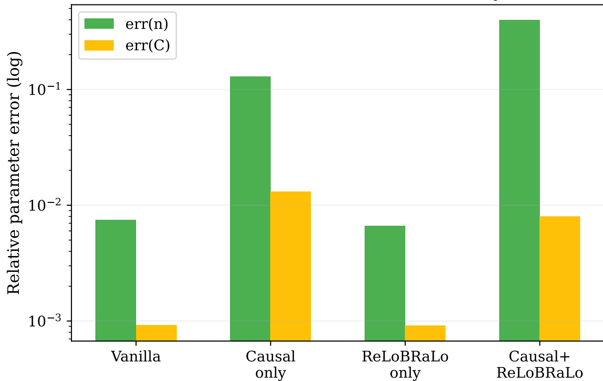
(b) Parameter identification accuracy
