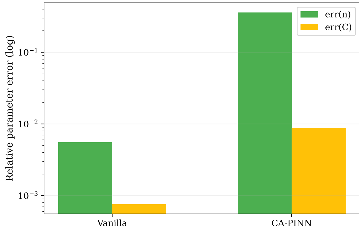
(b) Sparse data: parameter identification
