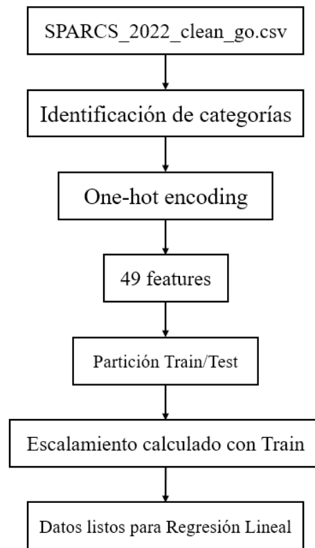
Figura 6. Flujo de preparación de datos para la Regresión Lineal
