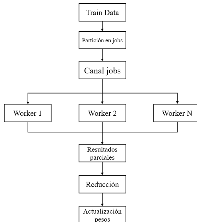
Figura 7. Arquitectura de la implementación concurrente en Go mediante el patrón Worker Pool
