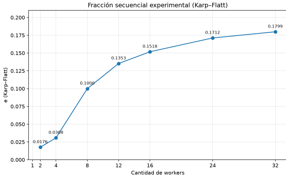
Figura 12. Fracción secuencial experimental (Karp–Flatt) según la cantidad de workers
