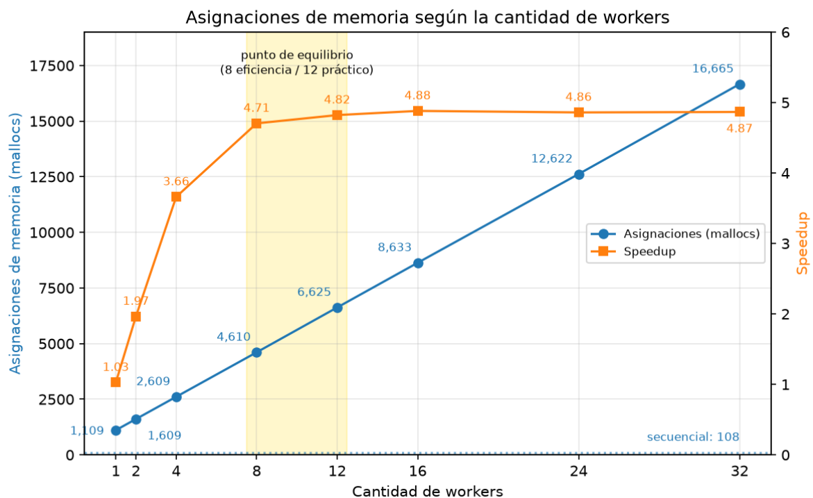
Figura 14. Asignaciones de memoria y speedup según la cantidad de workers
