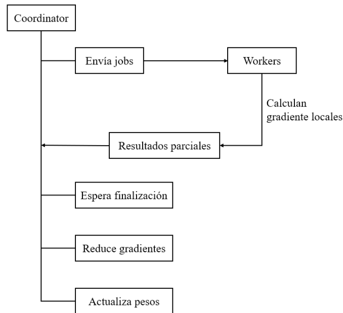
Figura 8. Flujo de sincronización de la implementación concurrente en Go
