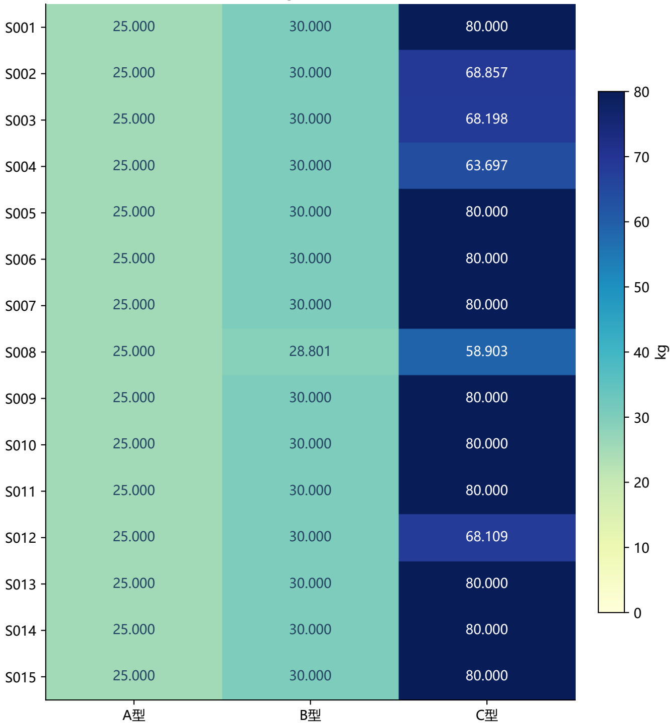
最大安全载荷 (kg) | 返航安全余量20%
