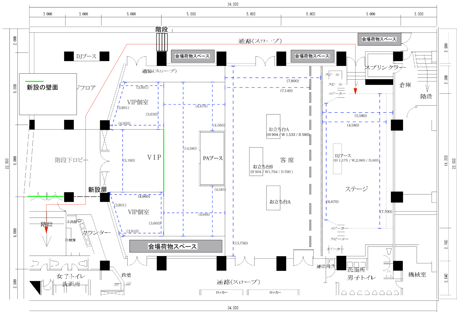
平面図 営業所平面図 S=1/100
