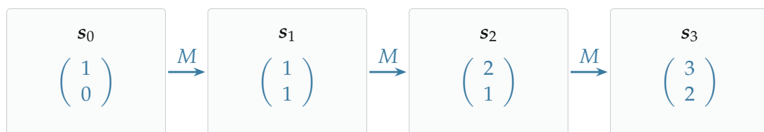
图 5.13: 斐波那契递推：每一步用同一个矩阵更新两项记忆。
