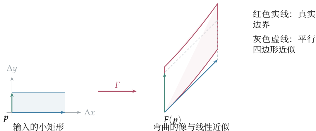
图 6.16: 小矩形在非线性变换后具有弯曲边界，灰色虚线平行四边形是局部线性近似。两侧分别采用位移坐标，图形已放大；蓝、绿箭头对应近似矩阵的两列，块越小，边界与线性近似越接近。
