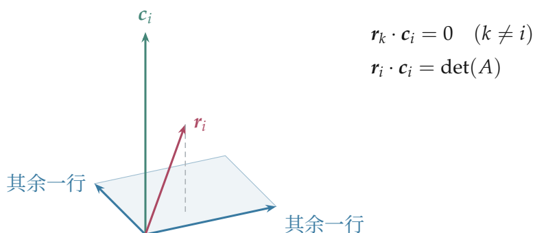
图 6.14: 固定其余两行, 先确定垂直方向, 再与第 i 行作点积。绿色向量 \mathbf{c}_i 垂直于蓝色底面; 红色的第 i 行一般不与它垂直, 因此能读出非零体积。
