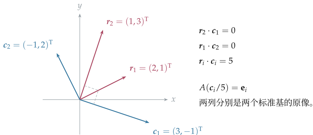
图 6.13: 红色两支箭头是矩阵 A = \begin{pmatrix} 2 & 1 \\ 1 & 3 \end{pmatrix} 的行向量, 蓝色两支是伴随矩阵的列。每支蓝色箭头垂直于另一行; 与对应行的点积都为 5, 除以 5 后成为逆矩阵的两列。
