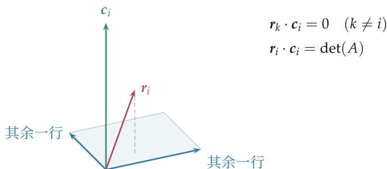
图 6.12: 固定其余两行, 先确定垂直方向, 再与第 i 行作点积。绿色向量 c_i 垂直于蓝色底面; 红色的第 i 行一般不与它垂直, 因此能读出非零体积。
