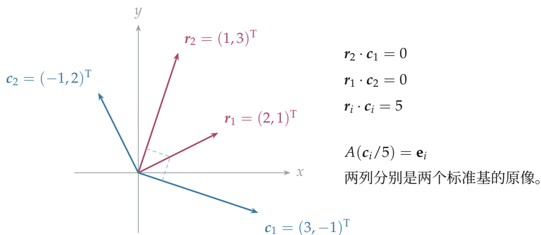
图 6.19: 红色两支箭头是矩阵 A = \begin{pmatrix} 2 & 1 \\ 1 & 3 \end{pmatrix} 的行向量, 蓝色两支是伴随矩阵的列。每支蓝色箭头垂直于另一行; 与对应行的点积都为 5, 除以 5 后成为逆矩阵的两列。
