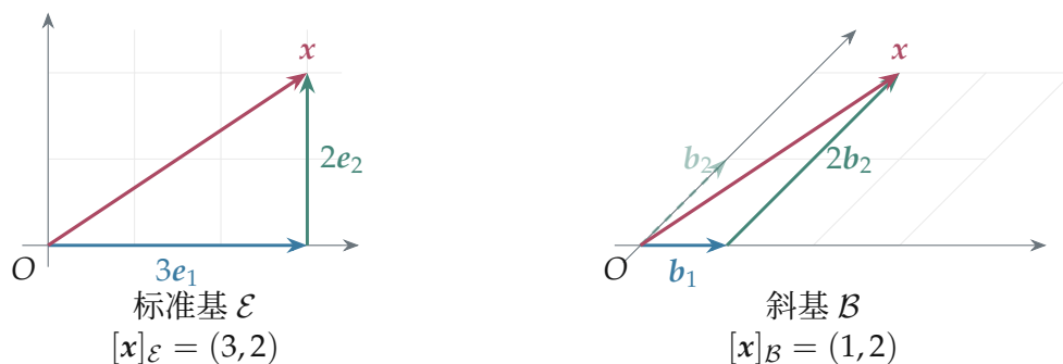
图 0.8: 同一个向量 (3, 2) 的两种分解。红色箭头不变, 所选的基与表示系数改变。
