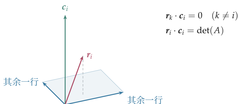
图 6.18: 固定其余两行，先确定垂直方向，再与第 i 行作点积。绿色向量 \mathbf{c}_i 垂直于蓝色底面；红色的第 i 行一般不与它垂直，因此能读出非零体积。
