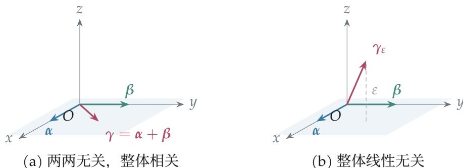
图 1.11: 三个向量的整体关系: 左图第三个向量仍在前两个张成的平面内, 整体相关; 右图第三个向量离开平面, 整体无关 (以 \varepsilon = 1 示意)。
