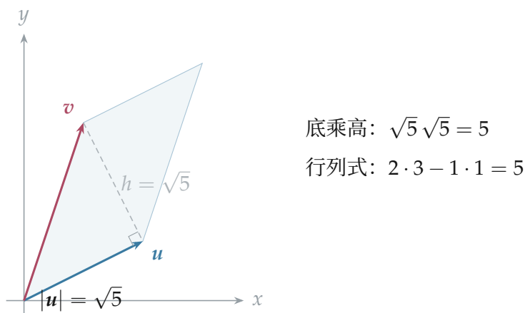
图 6.10: 底乘高与二阶行列式给出同一个面积。示例两条边为 (2, 1)^T 、 (1, 3)^T ，底长与高都为 \sqrt{5} ；灰色虚线为高，直角标记说明它垂直于底边，有向面积为 5。
