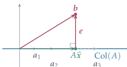
图 5.7b: 每一列都沿着蓝色直线; 最优输出到目标的误差, 与这些列全部垂直。
