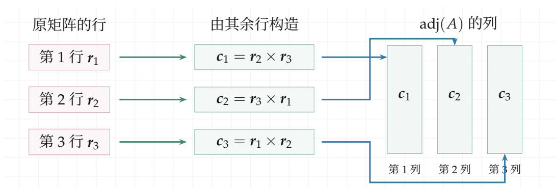
图 6.23: 左侧三行分别留下自己的位置，取另外两行的叉乘，得到中间的三支绿色法向量。右侧把它们放成伴随矩阵的三列，各列颜色和来源一一对应。这是 Shankar 的叉乘构造思路在本讲义记号下的呈现；转置排列来自行点列的运算要求。
