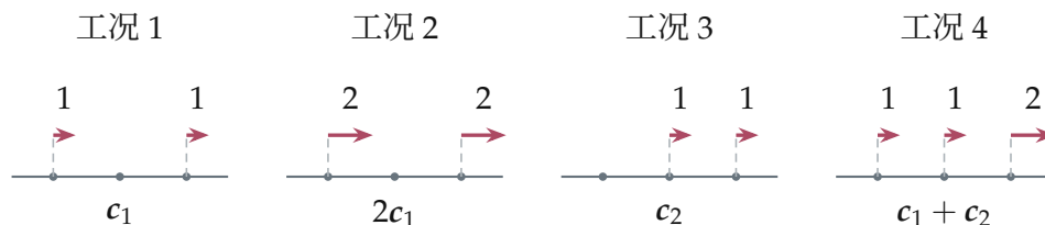
图 3.40: 从 CR 的列关系，读出工程工况之间的组合关系。
