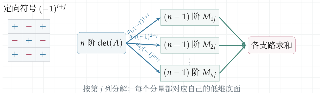
图 6.20: 左侧的正负号表由交换次数决定，右侧把第 j 列的各个元素分别配给一个低一阶行列式。每条支路都先取元素，再乘位置符号和对应余子式；最后求和。删去的位置不同，余下的低维底面也不同，不能只计算一个余子式反复使用。
