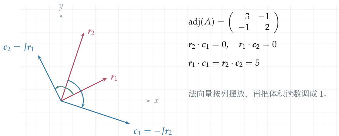
图 6.25: 红色箭头为矩阵 A = \begin{pmatrix} 2 & 1 \\ 1 & 3 \end{pmatrix} 的两行, 蓝色箭头为伴随矩阵的两列。第 2 行顺时针转 90^\circ 得到第 1 列, 第 1 行逆时针转 90^\circ 得到第 2 列; 两种方向不可混用。各列与对应行的点积都为 5, 除以 5 后满足 A(c_i/5) = e_i 。
