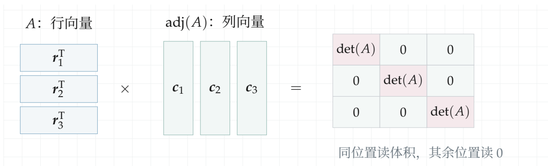
图 6.24: 左边每行与右边每列组成一个点积: 同位置的红色读数为 \det(A) , 其余绿色读数为 0。因此乘积只在主对角线留下体积。三阶图示对应式(6.75), 任意阶的证明使用完全相同的行列对应。
