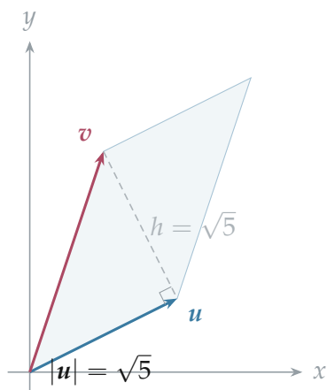
图 6.27: 底乘高与二阶行列式给出同一个面积。示例两条边为 (2, 1)^T 、 (1, 3)^T , 底长与高都为 \sqrt{5} ; 灰色虚线为高, 直角标记说明它垂直于底边, 有向面积为 5。
