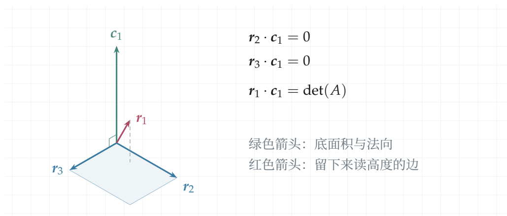
图 6.22: 蓝色两行张成底面, 绿色叉乘 c_1 = r_2 \times r_3 垂直于它们, 长度等于底面积。红色第 1 行一般斜向穿出底面, 与绿色法向量的点积为 \det(A) 。这支法向量属于“其余两行的正交补”, 不是第 1 行本身的垂直方向。
