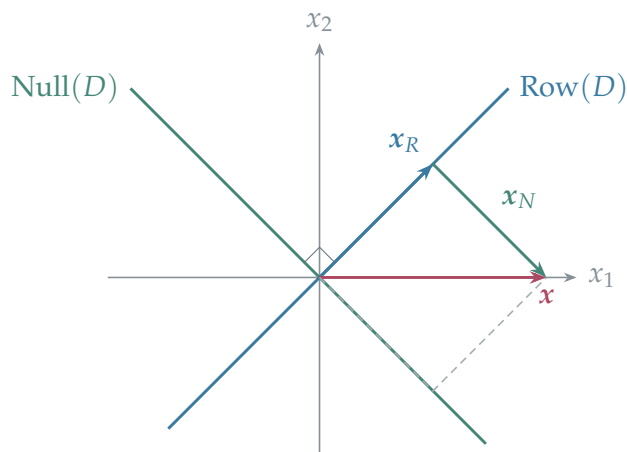
图 5.9: 输入端的正交直和: 行空间分量与零空间分量唯一相加。
