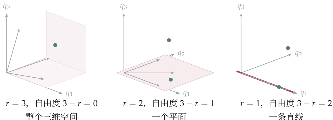
图 5.10d: 秩与可达目标的维数。为看清空间形状, 本图另取三个视频、三个特征的教学模型, 坐标轴 q_1, q_2, q_3 表示这三个特征。灰色箭头是视频向量, 淡红区域是列空间的有限示意, 绿点可达, 灰点不可达。三种库的秩依次为 3、2、1, 全部实数权重下的自由度依次为 0、1、2; 若限制非负权重或总和, 可执行目标还要取列空间中的相应部分。
