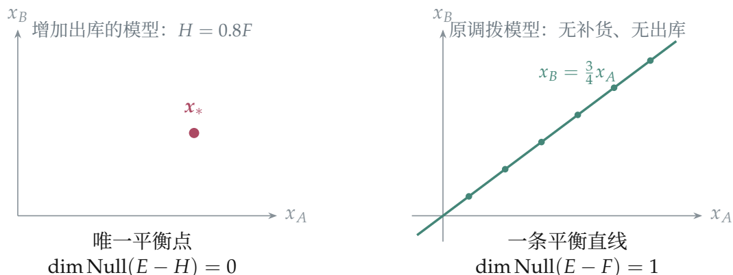
图 5.8d: 平衡状态的自由度: 有解时, 由 \text{Null}(E - F) 的维数决定。
