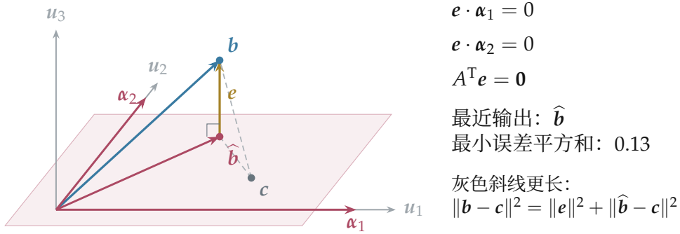
图 5.10e: 最小二乘的几何意义。蓝色目标不在红色列空间内，红色垂足 \hat{b} 是能达到的最近输出，黄色残差属于左零空间。坐标轴仍沿图 5.10b 的三个方向，灰色虚线连接目标与另一可达点 c 。直角标记和 A^T e = 0 对应式(5.135)；换用 c 会多出式(5.136)中的一个非负平方。本图仍是四维输出空间的三维截面，不把整个左零空间误画成一条线。
