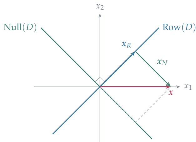
图 5.8: 输入端的正交直和: 行空间分量与零空间分量唯一相加。
