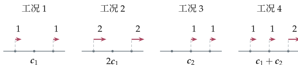
图 3.36: 从 CR 的列关系，读出工程工况之间的组合关系。
