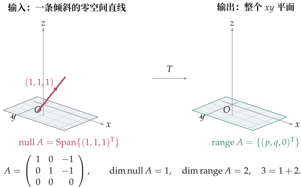
图 4.10: 零空间可以是一条不沿坐标轴的直线。
