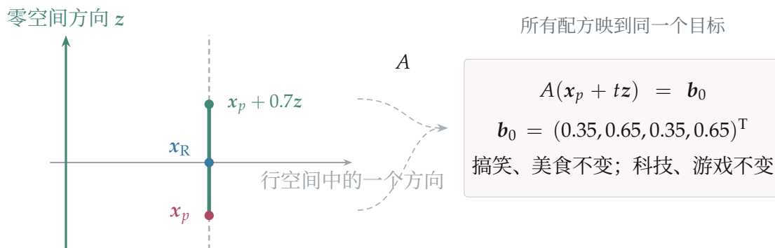
图 5.10c: 沿零空间移动，合成特征不变。左图取权重空间的二维截面，横向沿行空间中 x_R 的方向，纵向沿绿色零空间方向 z 。红点 x_p 、绿点 x_p + 0.7z 与蓝点 x_R 都属于式(5.127)，右侧只得到同一个四维目标。深绿线段满足本例的非负权重限制，灰色延长线属于全部实数解；不变的是合成特征，实际视频配方可以不同。
