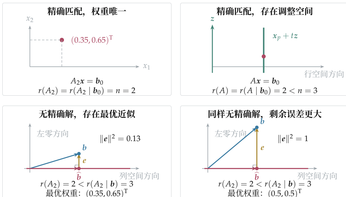
图 5.10g: 解的结构与推荐决策。上排画权重空间：只用前两列时，目标 b_0 的权重唯一；加入第三列后，全部解沿绿色零空间方向排成直线。下排画输出空间的二维截面，横向沿列空间，纵向沿左零空间；两个例子均用列无关的 A_2 = (\alpha_1 \alpha_2) ，所以最优权重唯一，黄色线段是不可消除的残差。右下目标 (1, 0, 0, 1)^T 的最小误差平方和为 1，大于本节目标的 0.13；它仍属无精确解的情形，不是第四种代数解类型。较大误差提示检查内容覆盖、特征表示和评价尺度，不能只靠继续调同一组权重解决。
