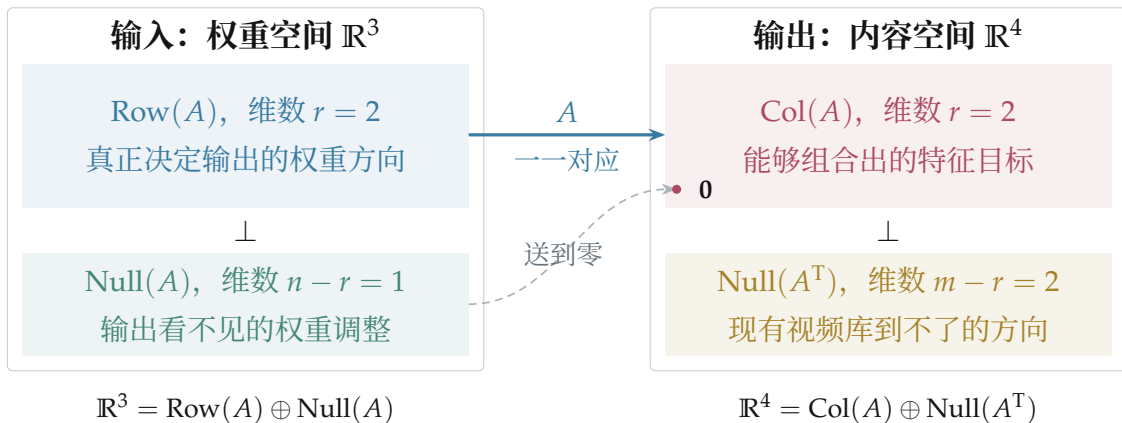
图 5.10a: 推荐模型的四个基本子空间。左框是三维权重空间，右框是四维内容特征空间，二者不能混为一谈。蓝色行空间一一映到红色列空间，绿色零空间被送到零；黄色左零空间记录不可达方向。本例四块的维数依次为 2、1、2、2，正交符号表示两端各自的互补关系。
