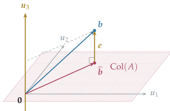
图 5.10b: 输出端的可达部分与不可达部分。红色平面表示列空间，蓝色箭头表示目标，黄色箭头表示残差，灰色虚线辅助辨认分解。坐标轴 u_1, u_2 沿列空间， u_3 沿一个左零空间方向，对应式(5.129)。本例输出为四维，左零空间也有二维；图只画 \text{Span}\{\alpha_1, \alpha_2, e\} 的三维截面，未画出的另一个左零方向仍然存在。
