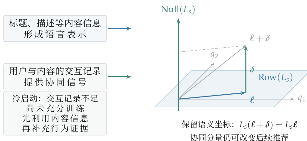
图 5.10f: 把语义约束与协同学习分开。左侧两条信息通路分别来自内容文本与交互记录，灰色卡片提醒冷启动首先是证据不足。右侧画式(5.140)的理想化三维截面：蓝色平面是保留语义的行空间，绿色方向是该语义作用的零空间，灰色总向量含两类分量。AlphaFuse 在弱语义方向学习 ID 表示；这些方向在实际方法中包括按阈值选择的近似零方向。图中不把新用户误画成权重空间里的一个点，也不把保留语义等同于全部推荐分数不变。
