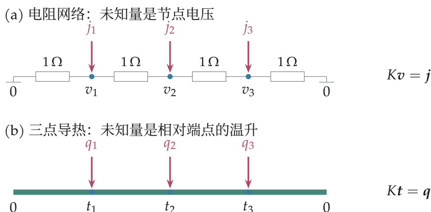
图 3.31: 结构响应、电路电压与稳态温度，都能形成“固定矩阵、变化输入”的任务。
