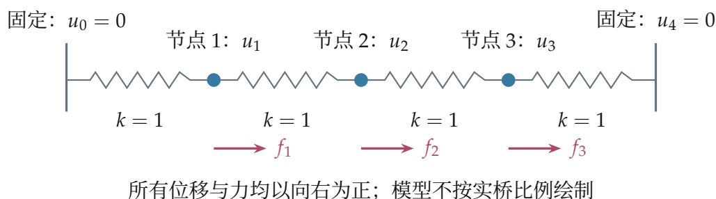
图 3.24: 从真实桥梁的多工况问题，抽取一个可手算的三节点连接模型。
