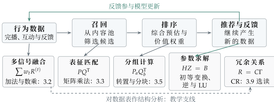
图 3.38: 推荐系统的公开流程，与本章五组矩阵运算的联系。
