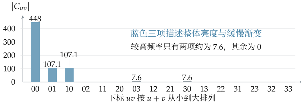
图 4.21: 本例的大系数集中在左侧的三个低频位置。
