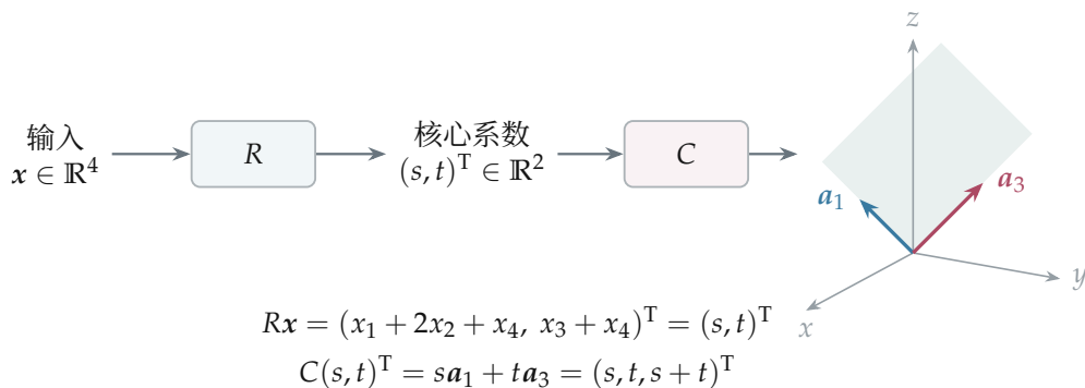
图 3.36: CR 分解先提取核心方向的组合系数，再把系数还原为输出。例题中两个核心列张成三维空间内的平面 z = x + y 。
