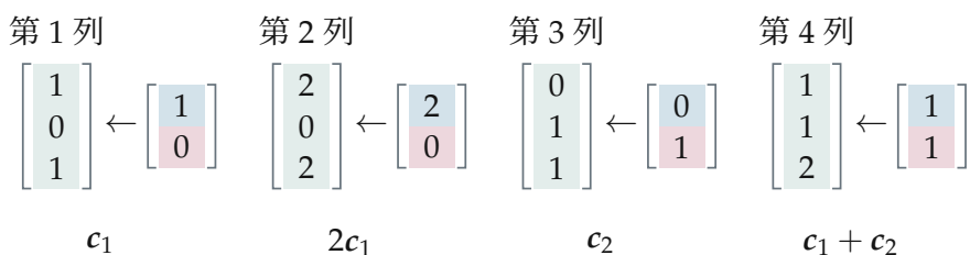
图 3.34: 逐列重建: R 的每一列都是一张“两种方向如何配比”的记录。
