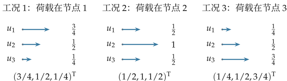
图 3.29: 同一个连接模型, 三种荷载位置, 三组位移响应。
