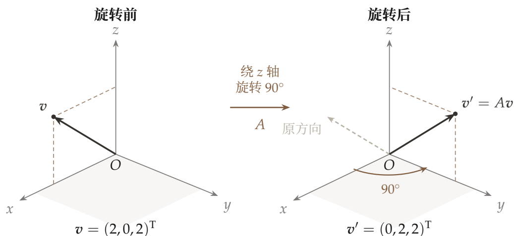
图 4.0b: 固定同一组 \mathbb{R}^3 坐标轴，向量绕 z 轴旋转。浅色虚线只保留原方向作比较；实线箭头的终点发生了变化。
