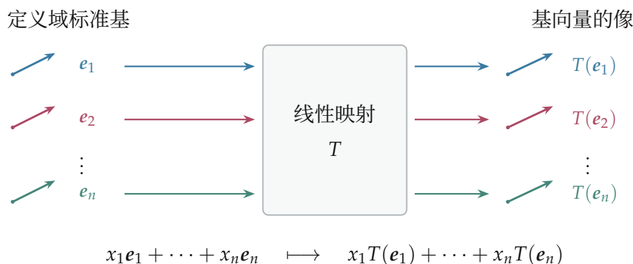
图 3.2: 线性映射的确定性。只要确定了每个基向量的像，整个空间中任意向量的像都随之唯一确定。
