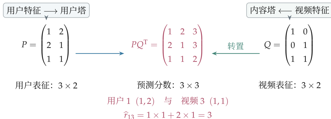
图 3.39: 两端分别产生表征，一次矩阵乘法汇集全部配对分数。
