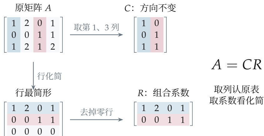
图 3.33: CR 的两条取材路线: 原矩阵给出方向, 行最简形给出系数。
