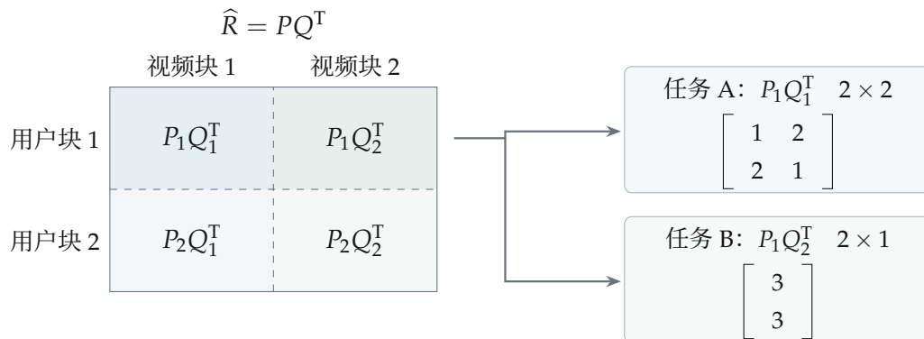
图 3.40: 按用户和视频分块，各块可以分别计算，再按原位置拼接。
