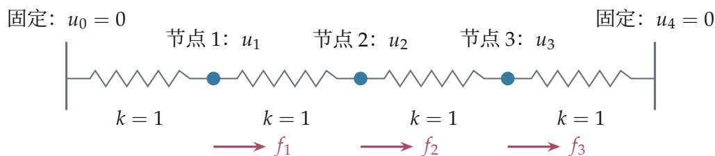
图 3.29: 从真实桥梁的多工况问题，抽取一个可手算的三节点连接模型。
