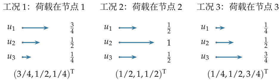
图 3.30: 同一个连接模型，三种荷载位置，三组位移响应。
