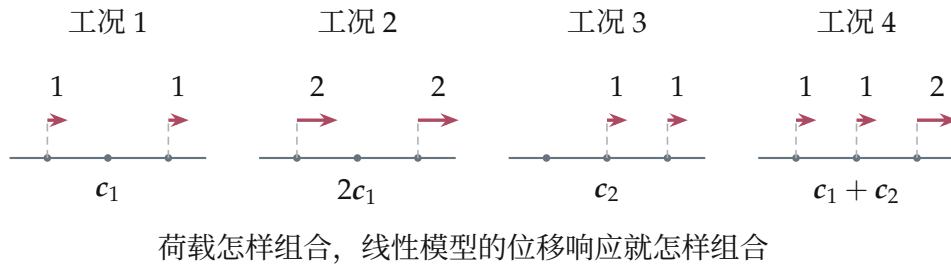
图 3.36: 从 CR 的列关系，读出工程工况之间的组合关系。
