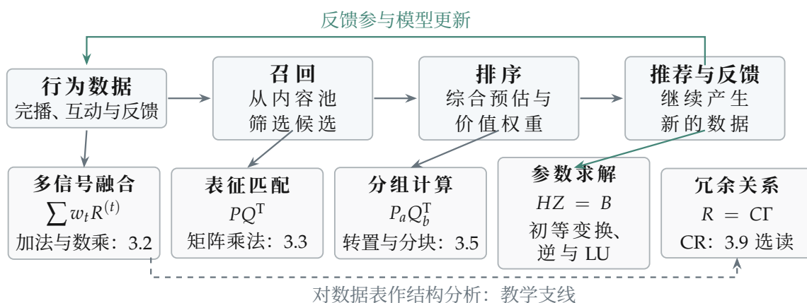
图 3.37: 推荐系统的公开流程，与本章五组矩阵运算的联系。
