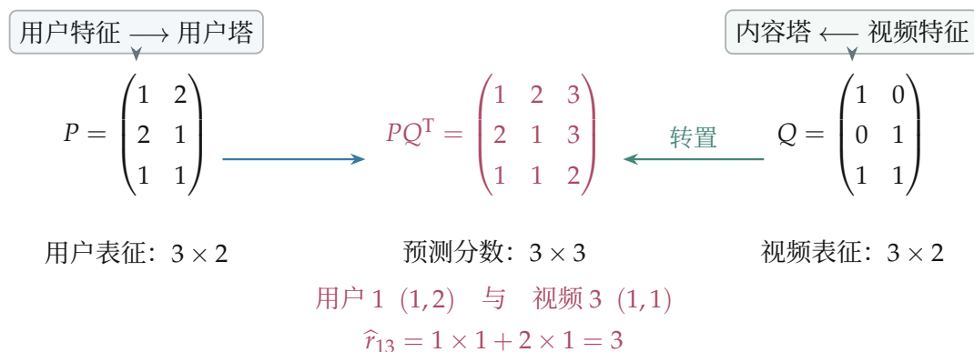
图 3.38: 两端分别产生表征，一次矩阵乘法汇集全部配对分数。
