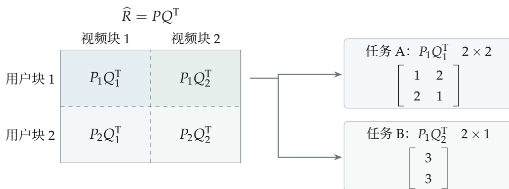
图 3.39: 按用户和视频分块，各块可以分别计算，再按原位置拼接。
