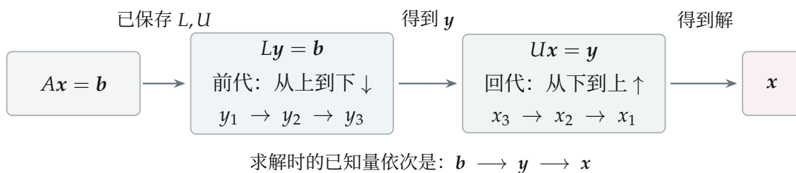
图 3.25: 先解下三角方程, 再解上三角方程; 箭头同时标出求解顺序与逐行计算方向。
