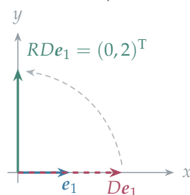
图 3.15: 交换复合的先后次序，会改变结果。两条路线从同一个输入出发，最终的纵向长度不同。
