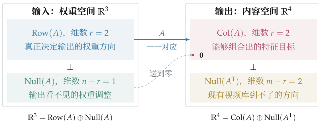
图 5.10a: 推荐模型的四个基本子空间。左框是三维权重空间，右框是四维内容特征空间，二者不能混为一谈。蓝色行空间一一映到红色列空间，绿色零空间被送到零；黄色左零空间记录不可达方向。本例四块的维数依次为 2、1、2、2，正交符号表示两端各自的互补关系。
