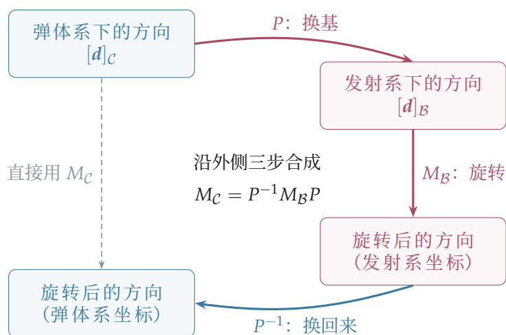
图 4.17e: 姿态矩阵的相似变换环: M_C = P^{-1}M_BP 。
