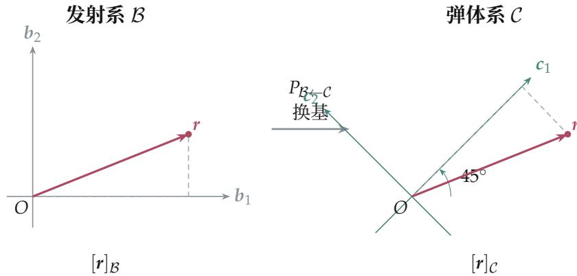
图 4.17c: 同一个位置向量 r , 在发射系 B 与弹体系 C 下的坐标不同, 中间由过渡矩阵 P_{B \leftarrow C} 换算。
