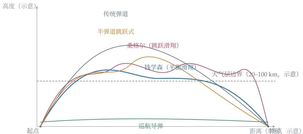
图 4.17a: 五种弹道共享同一个起点和终点，区别在于再入段之后的飞行方式。钱学森弹道的独特之处在于：再入后不再飞出大气层，而是贴着大气层边缘做平滑滑翔。
