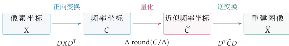
图 4.18: 换基可逆，量化丢失细节，再用逆变换重建。
