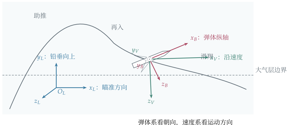
图 4.17b: 钱学森弹道的助推、再入、滑翔三个阶段，以及发射系（蓝）、弹体系（红）、速度系（绿）三组坐标架。
