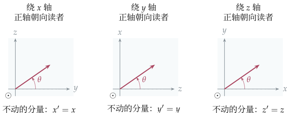
图 4.6b: 三维旋转的三个二维截面。绕 x, y, z 轴时，分别在 (y, z) 、 (z, x) 、 (x, y) 有序平面中使用同一个二维旋转模板。
