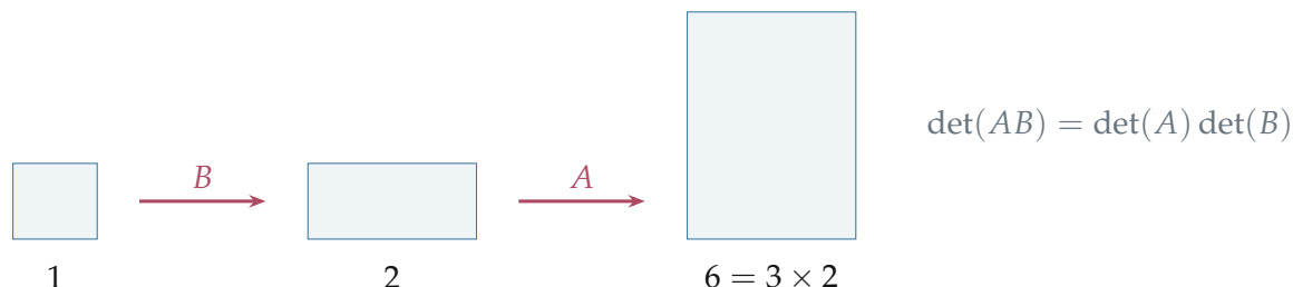
图 6.12: 复合变换的面积倍率相乘。单位正方形先经 B = \text{diag}(2, 1) , 再经 A = \text{diag}(1, 3) , 面积依次为 1、2、6; 此例两步都保持方向。
