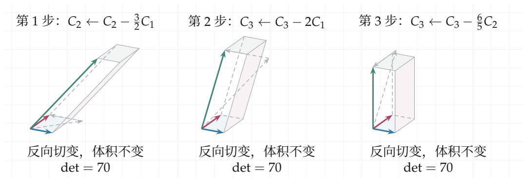
图 6.15: 三栏分别画出三次列倍加后的平行六面体，采用相同的坐标比例；蓝、红、绿箭头表示当前的三列，灰色虚线箭头表示本步操作前被调整的那条边。沿已有边撤销切变，斜盒子逐次变成沿坐标轴排列的长方体。三次操作均保持体积，行列式始终为 70。
