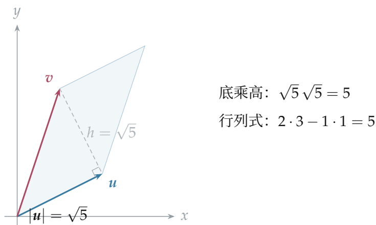
图 6.19: 底乘高与二阶行列式给出同一个面积。示例两条边为 (2, 1)^T 、 (1, 3)^T ，底长与高都为 \sqrt{5} ；灰色虚线为高，直角标记说明它垂直于底边，有向面积为 5。
