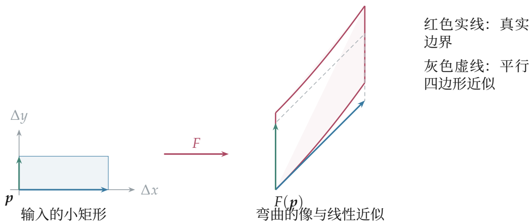
图 6.18: 小矩形在非线性变换后具有弯曲边界, 灰色虚线平行四边形是局部线性近似。两侧分别采用位移坐标, 图形已放大; 蓝、绿箭头对应近似矩阵的两列, 块越小, 边界与线性近似越接近。
