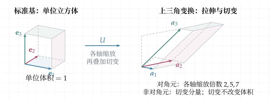
图 6.14: 左图是标准基围出的单位立方体，右图是矩阵 U = \begin{pmatrix} 2 & 3 & 4 \\ 0 & 5 & 6 \\ 0 & 0 & 7 \end{pmatrix} 的列向量围出的平行六面体，两图分别缩放排版。蓝、红、绿三条边的新增坐标分量依次为 2、5、7；灰色虚线标出非对角分量造成的偏移。切变改变形状而不改变有向体积，体积缩放因子为 2 \cdot 5 \cdot 7 = 70 。
