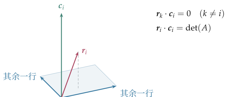
图 6.16: 固定其余两行，先确定垂直方向，再与第 i 行作点积。绿色向量 \mathbf{c}_i 垂直于蓝色底面；红色的第 i 行一般不与它垂直，因此能读出非零体积。
