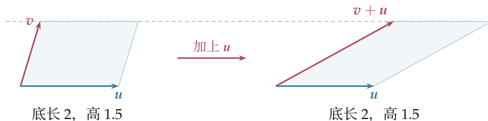
图 6.11: 向上边加上底边的倍数, 只让顶端横向移动。左、右两块平行四边形的底长与高都相同; 灰色虚线标出共同的高度, 因此有向面积相等。
