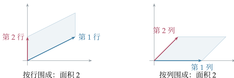
图 6.13: 同一矩阵 A = \begin{pmatrix} 2 & 1 \\ 0 & 1 \end{pmatrix} 的行与列围出不同形状的平行四边形, 但有向面积都为 2。转置不要求两幅图全等, 只保证行列式相等。
