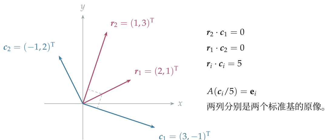
图 6.17: 红色两支箭头是矩阵 A = \begin{pmatrix} 2 & 1 \\ 1 & 3 \end{pmatrix} 的行向量, 蓝色两支是伴随矩阵的列。每支蓝色箭头垂直于另一行; 与对应行的点积都为 5, 除以 5 后成为逆矩阵的两列。
