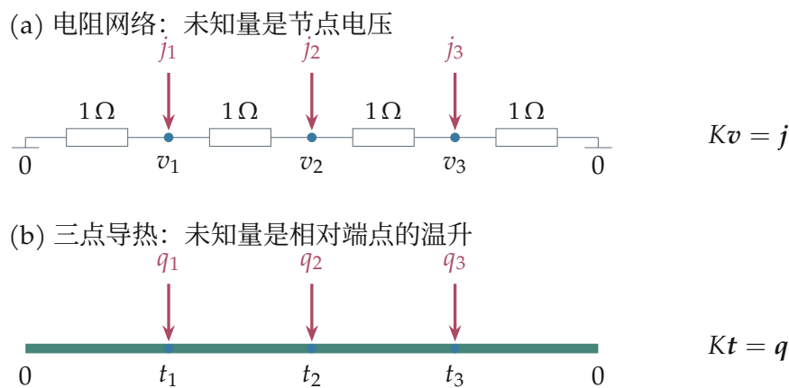
图 3.32: 结构响应、电路电压与稳态温度，都能形成“固定矩阵、变化输入”的任务。
