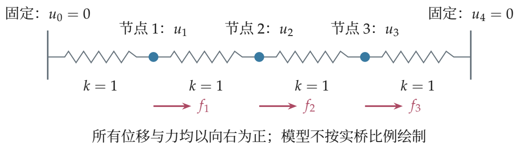
图 3.25: 从真实桥梁的多工况问题，抽取一个可手算的三节点连接模型。
