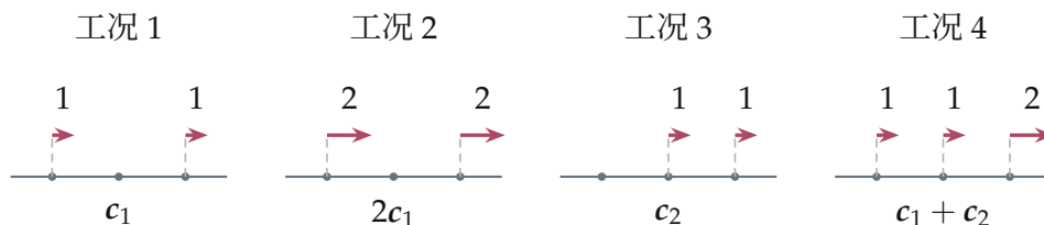
图 3.38: 从 CR 的列关系，读出工程工况之间的组合关系。
