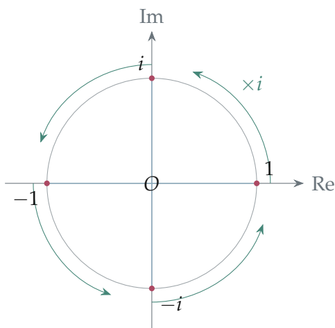
图 A.5: 四次单位根 1, i, -1, -i 均匀分布在单位圆上。每次乘以 i 都逆时针转过 \pi/2 ，四次以后回到原处。
