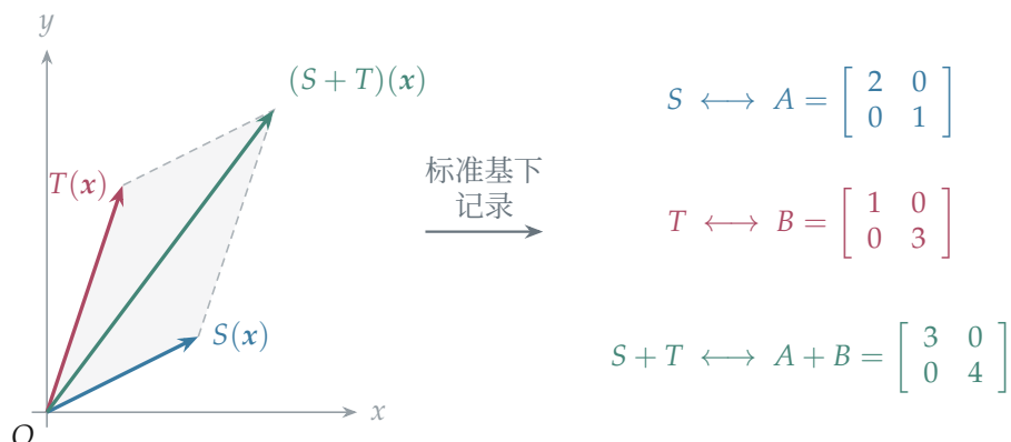
图 3.7: 映射的加法对应矩阵的加法。左图以输入 x = (1, 1)^T 为例，两个输出按平行四边形法则相加；右图记录相应矩阵。
