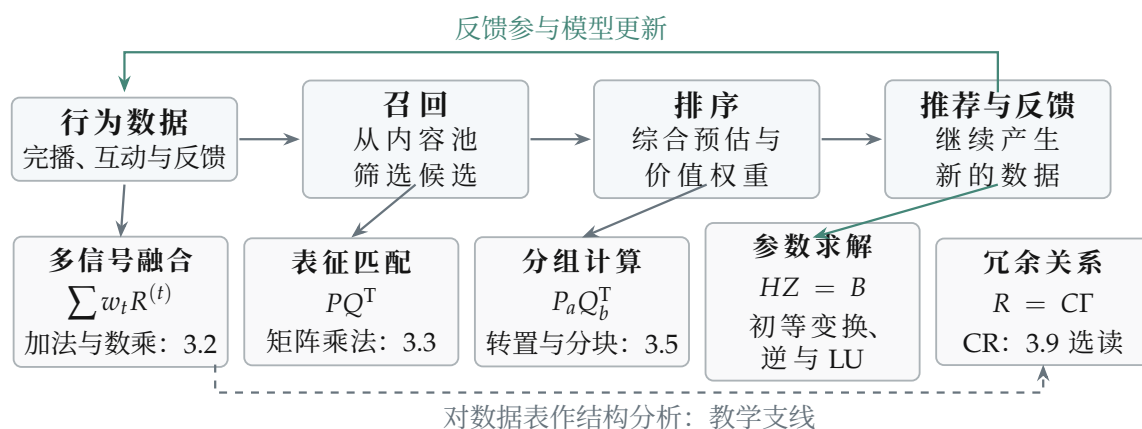
图 3.39: 推荐系统的公开流程，与本章五组矩阵运算的联系。
