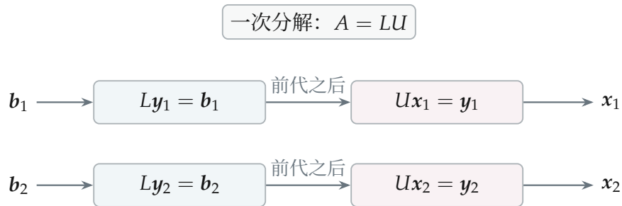
图 3.31: 分解只针对 A 做一次；每个新的右端项都复用同一个 L 与 U 。
