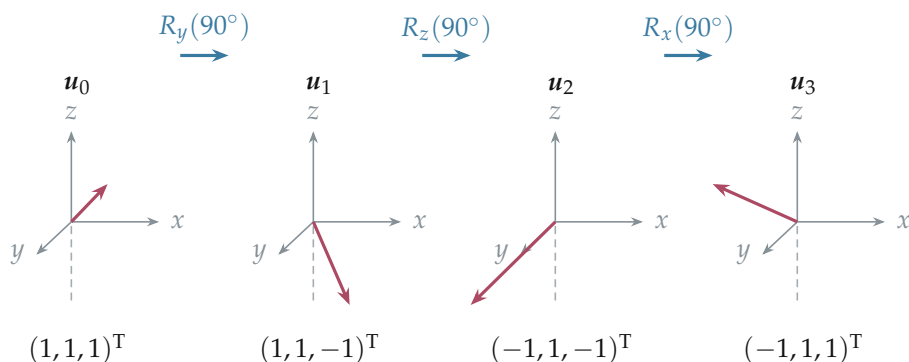
图 4.17g: 绕固定轴依次旋转, 与从右向左作用的矩阵乘积对应。图中三个角均取 90^\circ , 只为跟踪坐标变化。
