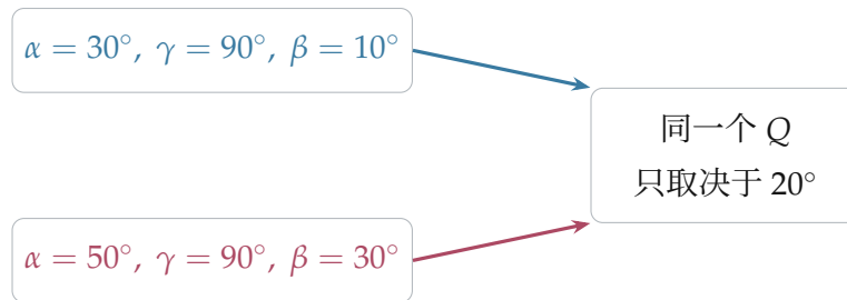
图 4.17i: 不同角度记录可以给出同一个旋转矩阵。当中间角为 90^\circ 时，本例中的矩阵只依赖差角 \alpha - \beta 。
