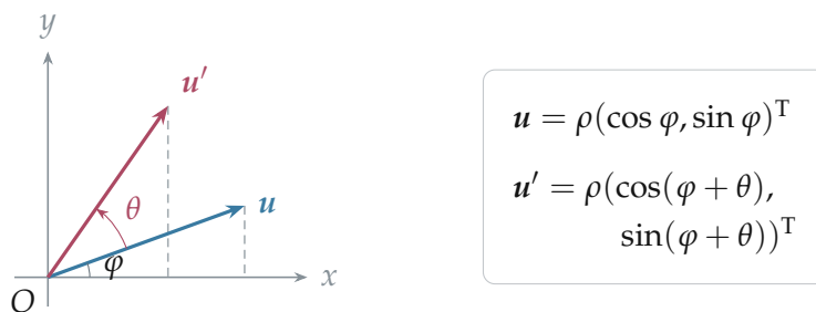
图 4.17c: 平面旋转的推导：长度 \rho 不变，有向角从 \varphi 变成 \varphi + \theta ，再用两角和公式展开坐标。
