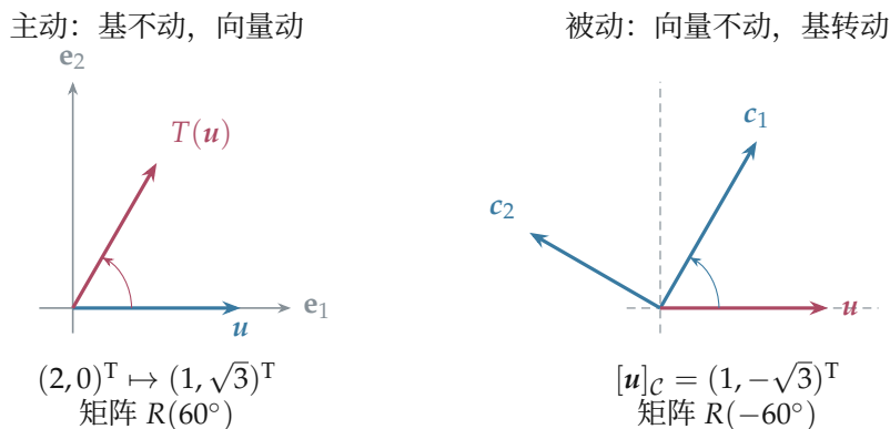
图 4.17e: 主动旋转与被动旋转。左图改变物理向量，右图保持向量不动、改变描述它的基。
