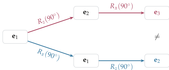
图 4.17h: 同样两个旋转, 次序不同, 终点不同。上、下两条路线都从 \mathbf{e}_1 出发, 分别到达 \mathbf{e}_3 与 \mathbf{e}_2 。
