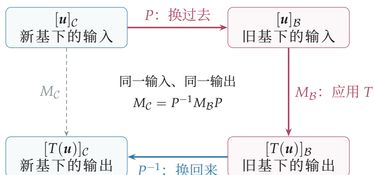
图 4.17j: 同一旋转的两条计算路线：先换基、应用旋转、换回来，等价于直接使用新基下的矩阵。
