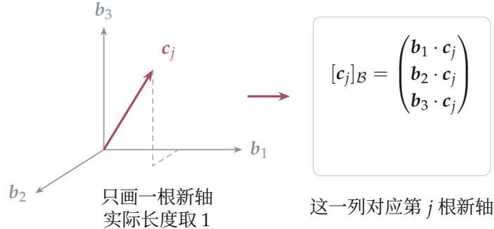
图 4.17f: 从一根新轴到矩阵的一列。三个方向余弦给出新轴在旧基下的三个分量, 三根新轴并列便得到 P 。
