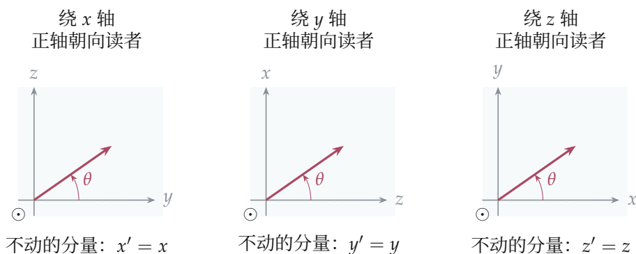
图 4.17d: 三维旋转的三个二维截面。绕 x, y, z 轴时，分别在 (y, z) 、 (z, x) 、 (x, y) 有序平面中使用同一个二维旋转模板。
