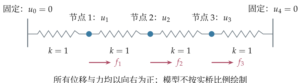
图 3.29: 从真实桥梁的多工况问题，抽取一个可手算的三节点连接模型。
