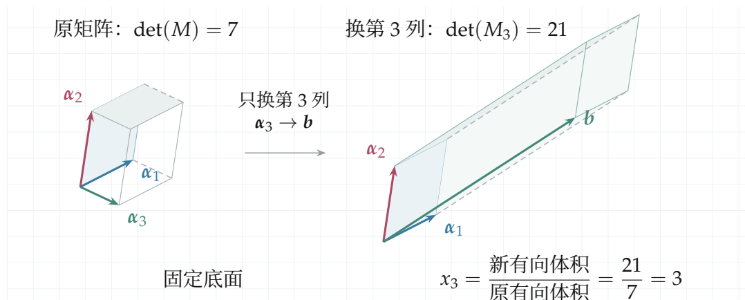
图 6.31: 两图保留相同的蓝、红底边, 即本例的第 1、2 列; 右图只把绿色第 3 条边换成目标 b , 浅绿色侧面显示新盒子的伸展。两图使用同一三维投影和坐标比例, 原有定向体积为 7, 新定向体积为 21, 所以第 3 个组合系数为 3。替换的是一条边对应的列, 底面保持不变。
