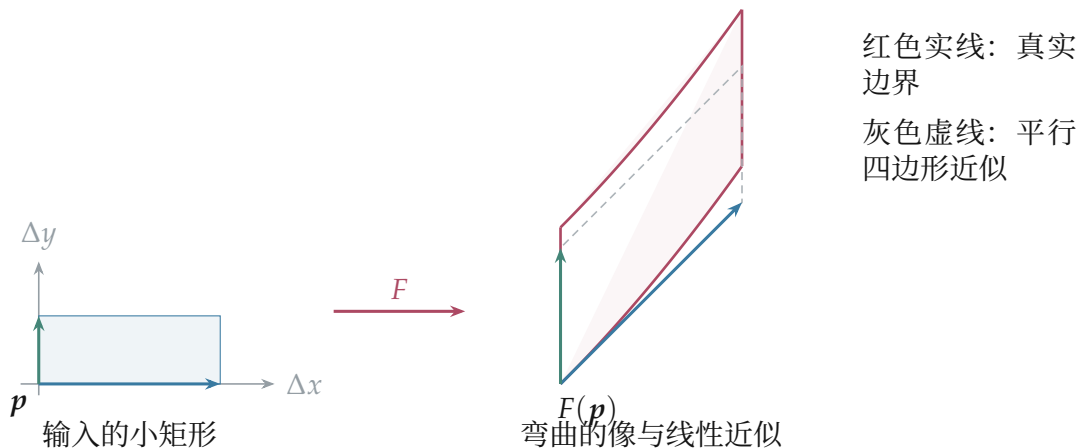
图 6.34: 小矩形在非线性变换后具有弯曲边界，灰色虚线平行四边形是局部线性近似。两侧分别采用位移坐标，图形已放大；蓝、绿箭头对应近似矩阵的两列，块越小，边界与线性近似越接近。
