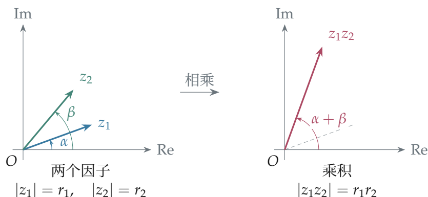
图 A.3: 复数乘法的极坐标解释。左图给出两个因子，右图给出乘积：长度变为 r_1 r_2 ，方向角变为 \alpha + \beta 。示意取 r_1 = 1.4 、 r_2 = 1.5 、 \alpha = \pi/9 、 \beta = 5\pi/18 。
