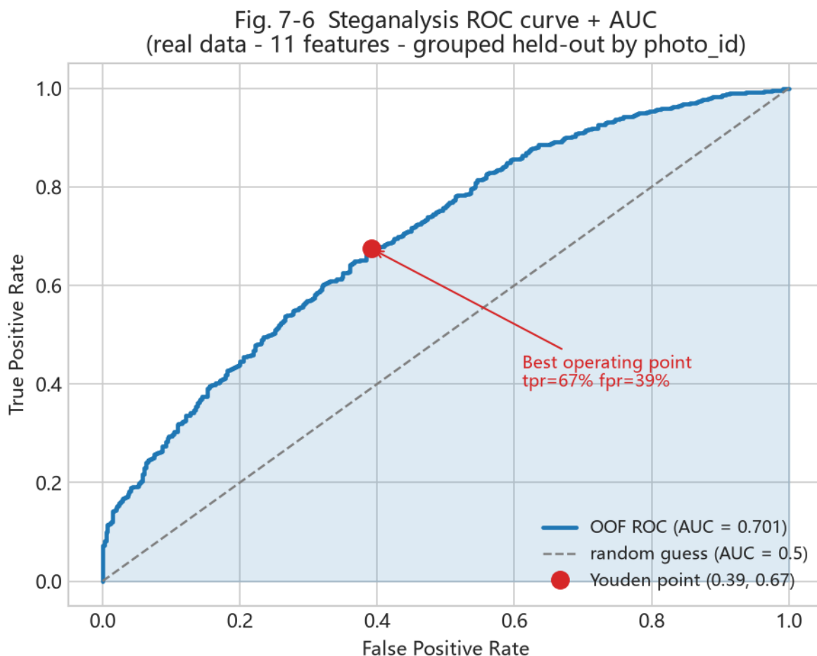
Figure 21: Fig. 7-6 ROC + AUC
