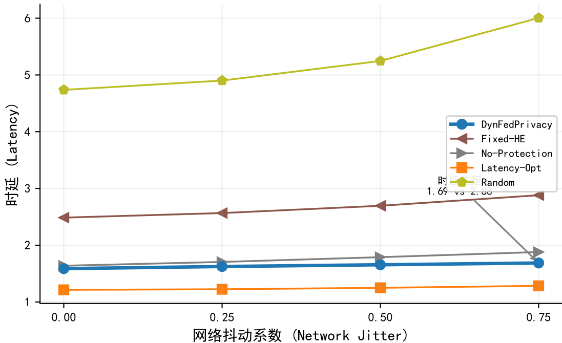
网络抖动对不同策略时延的影响
