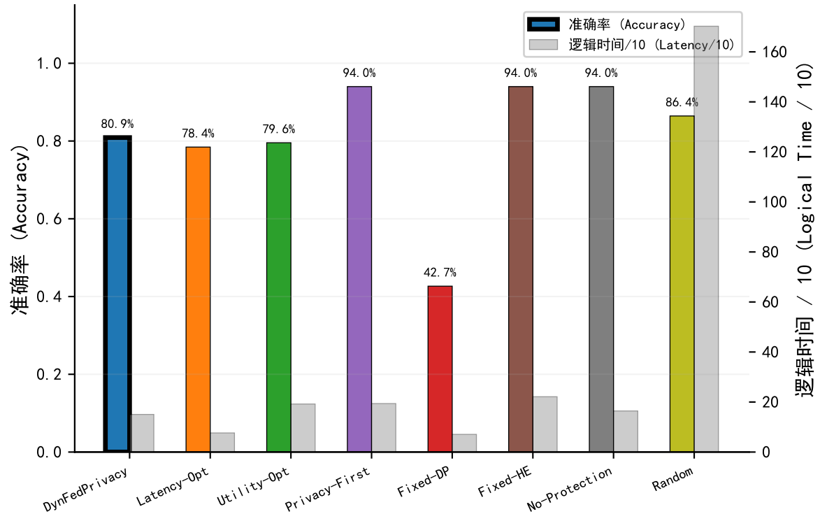
(b) 最终准确率与时延对比 Final Accuracy & Latency
