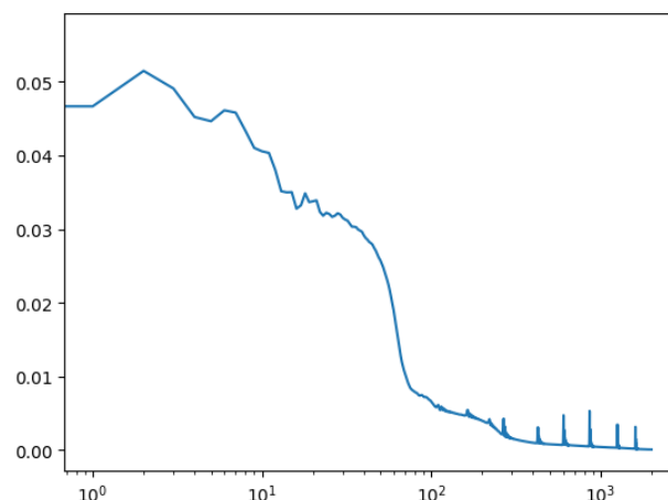
Рис. 2 – График обучения
