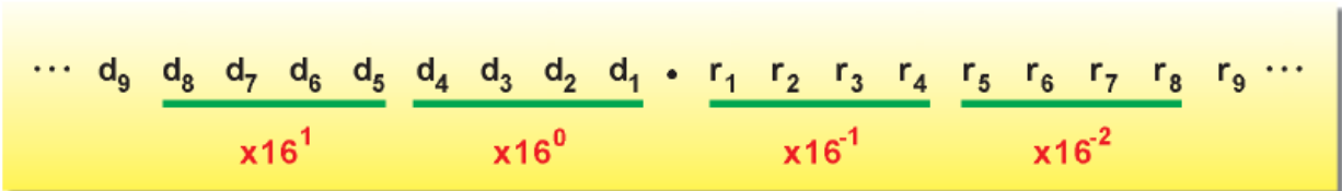
圖 2-7 二進位數換成十六進位數時，每四個位數合成一項
