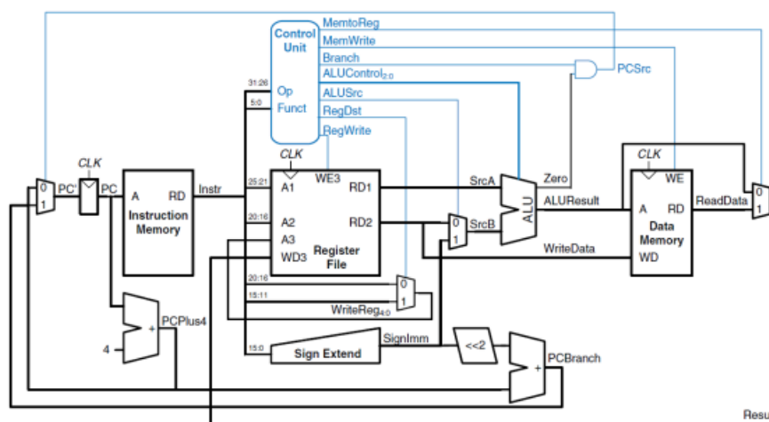
图 2.1 总体结构图
