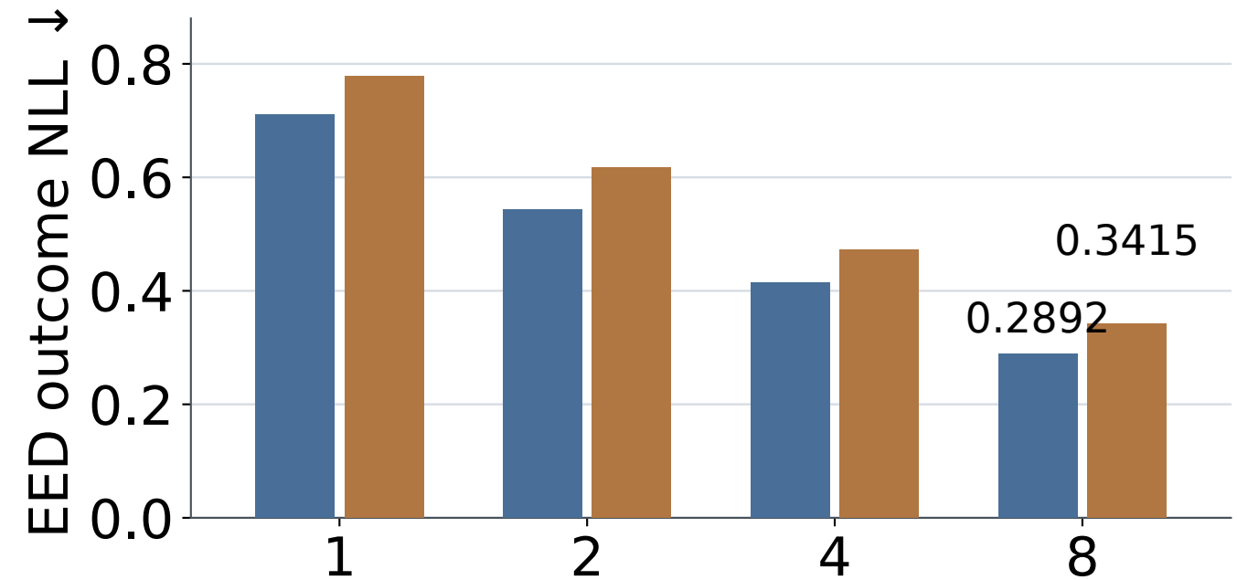
(b) CodeARC
