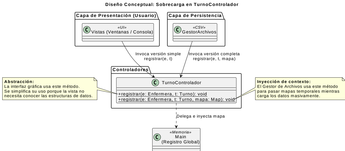
Figura 5.1: Diseño conceptual de la sobrecarga de métodos
