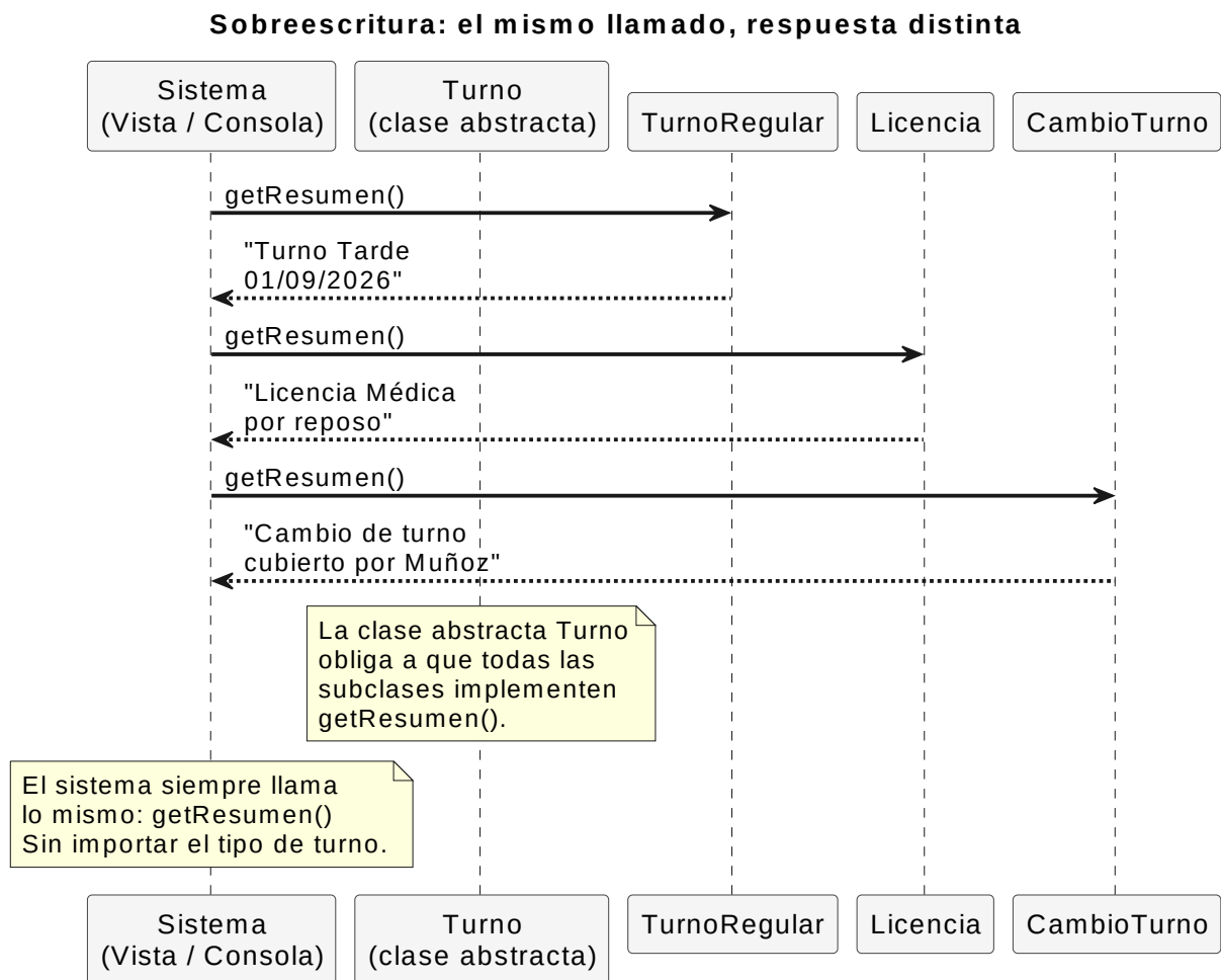
Figura 6.1: Diseño conceptual de la sobreescritura y el polimorfismo
