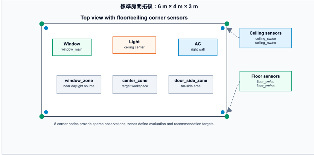
圖 3-3 房間感測器與目標區域配置。8 顆角落感測器、3 個主要區域與 3 個核心裝置共同構成單房間數位孿生的標準拓樸。
