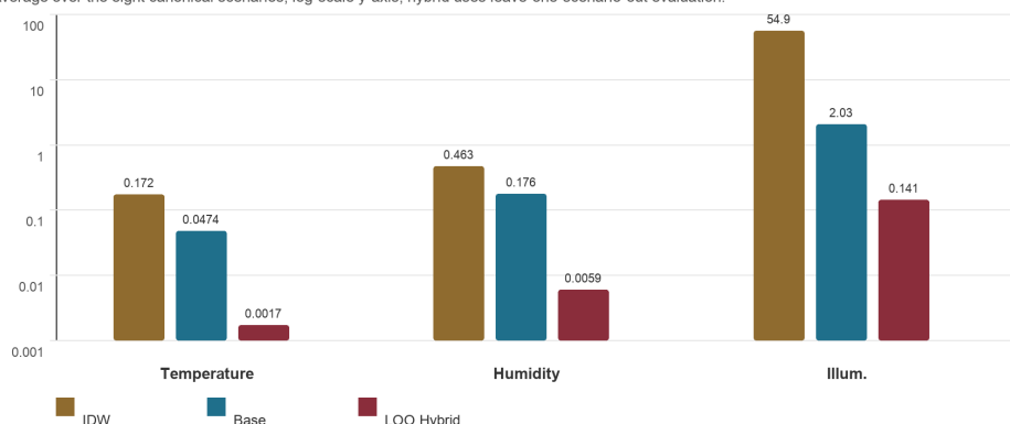
圖 5-5 IDW、base model 與 LOO hybrid residual correction 的平均 field MAE 比較。圖中使用 log-scale y-axis，數值為 8 組標準情境平均。
