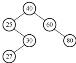
二叉树 T_1
