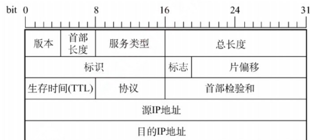
图1 IP分组头结构
