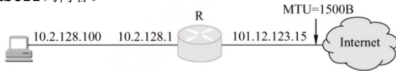
图1 网络拓扑
