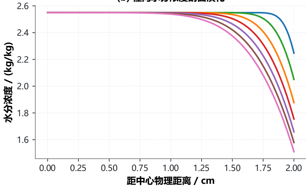
(b) 径向水分浓度剖面演化
