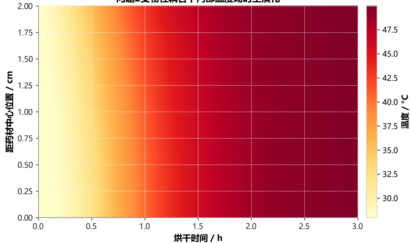
问题2变物性耦合下内部温度场时空演化
