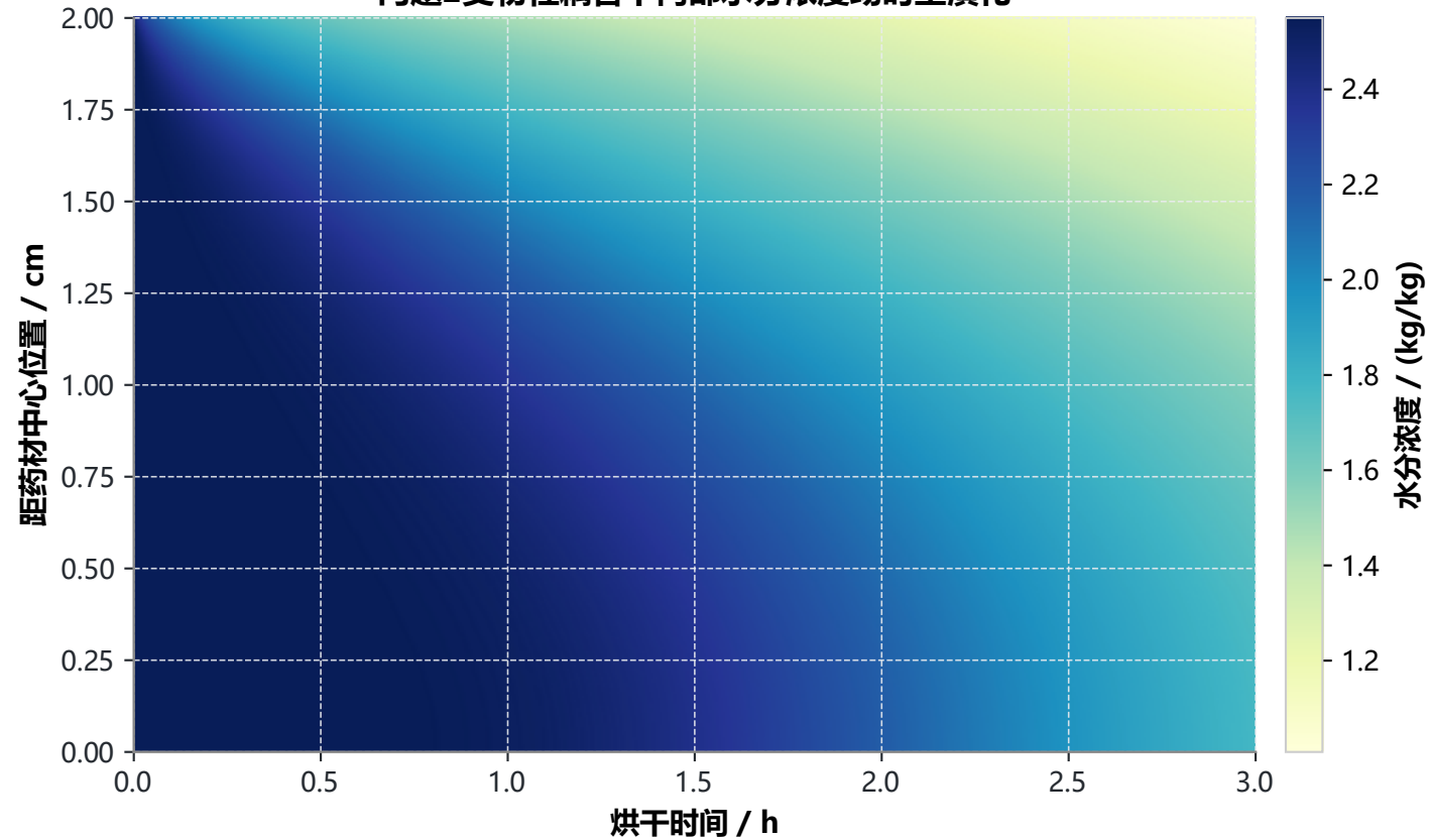
问题2变物性耦合下内部水分浓度场时空演化
