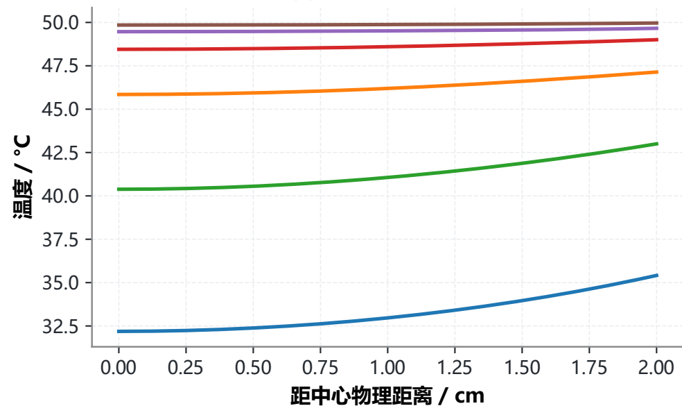
(a) 径向温度剖面演化
