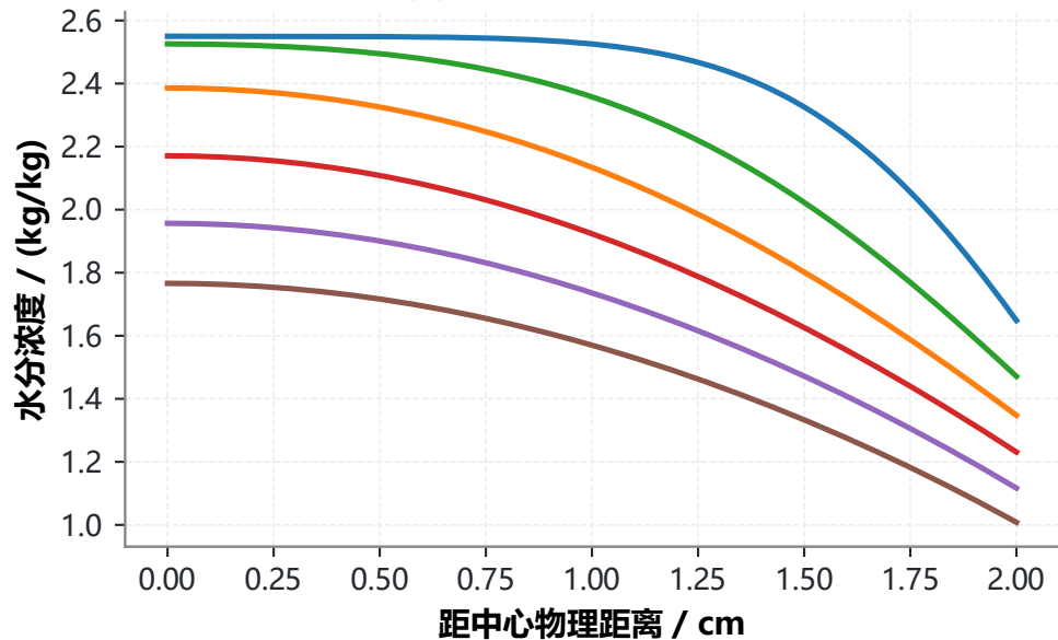
(b) 径向水分浓度剖面演化
