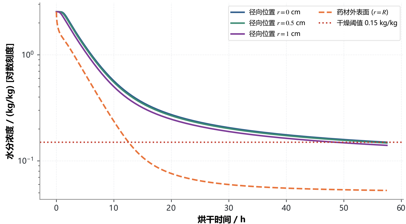
问题3固定截面模型各径向测点水分浓度衰减历程
