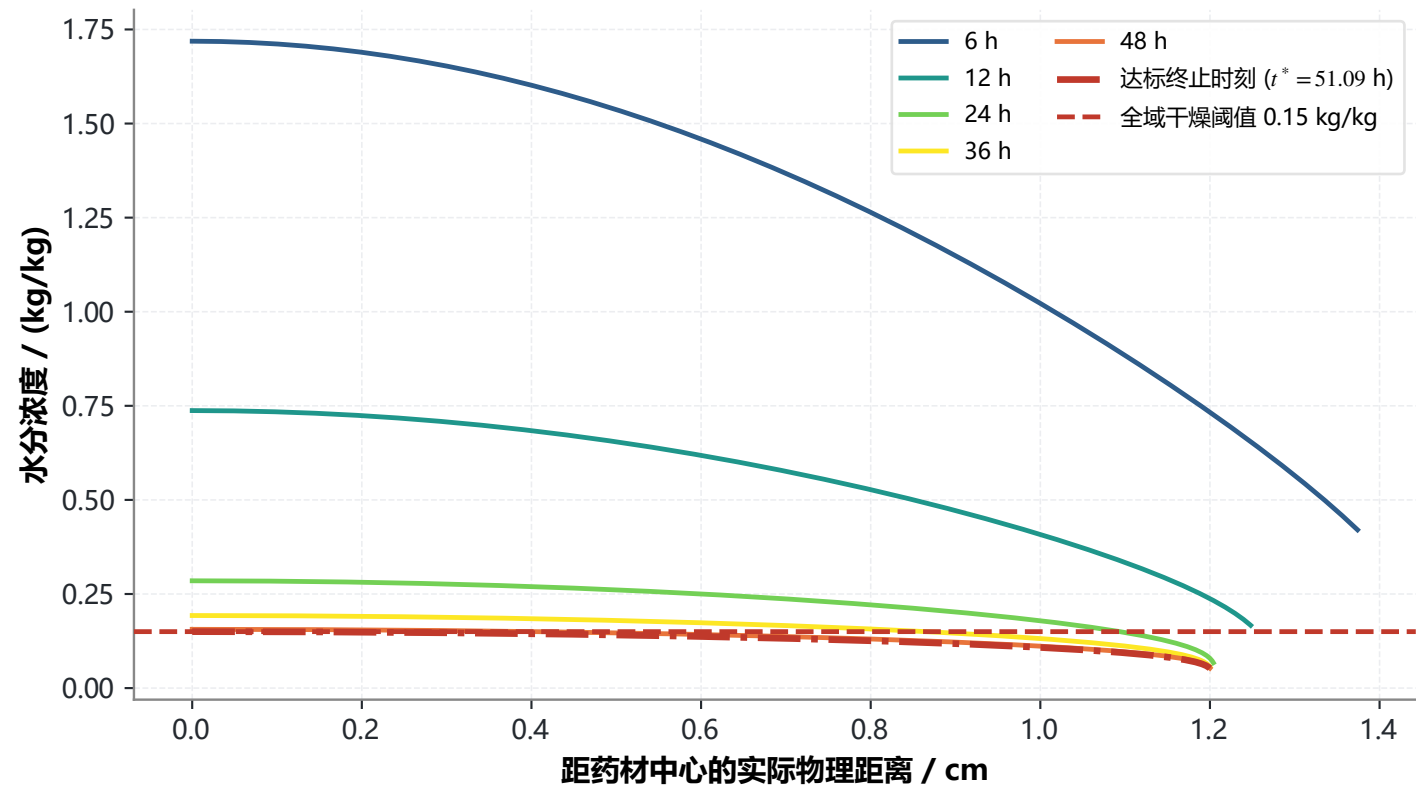
问题4 (收缩动边界) 真实物理尺度下的水分剖面演化
