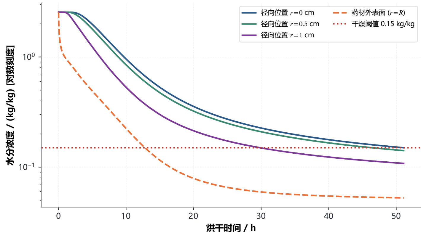
问题4收缩动边界模型各径向测点水分浓度衰减历程
