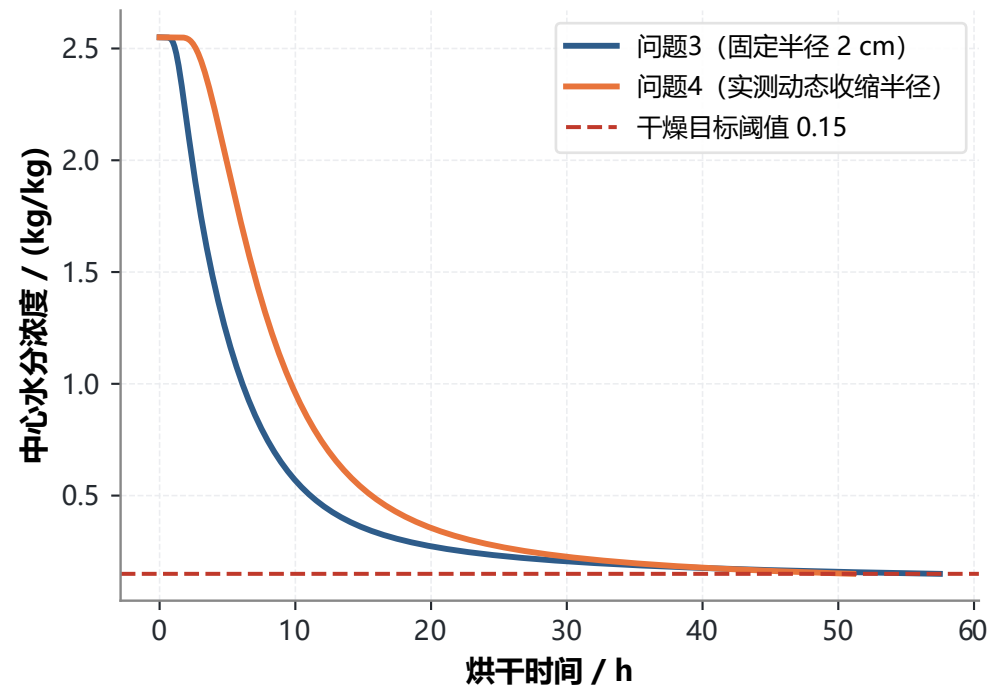
(a) 中心水分浓度衰减历程对比
