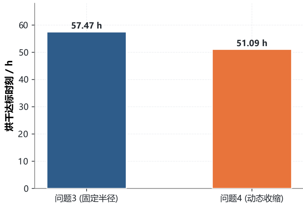
(b) 烘干所需总时长对比
