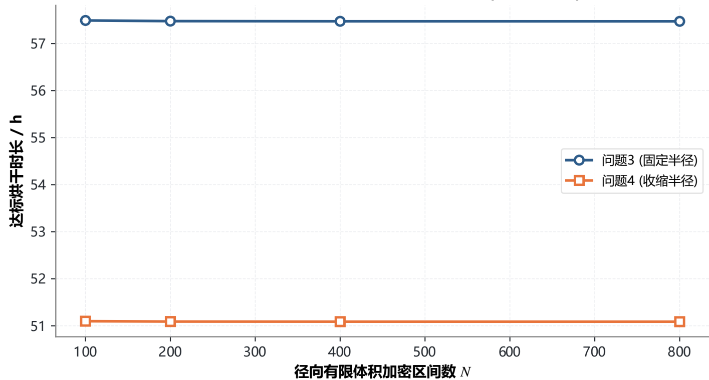
有限体积网格加密下的达标时刻单调收敛性（二阶表观阶）
